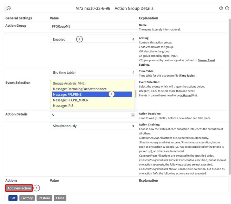
Fig. 32: Configuración de un grupo de acciones
