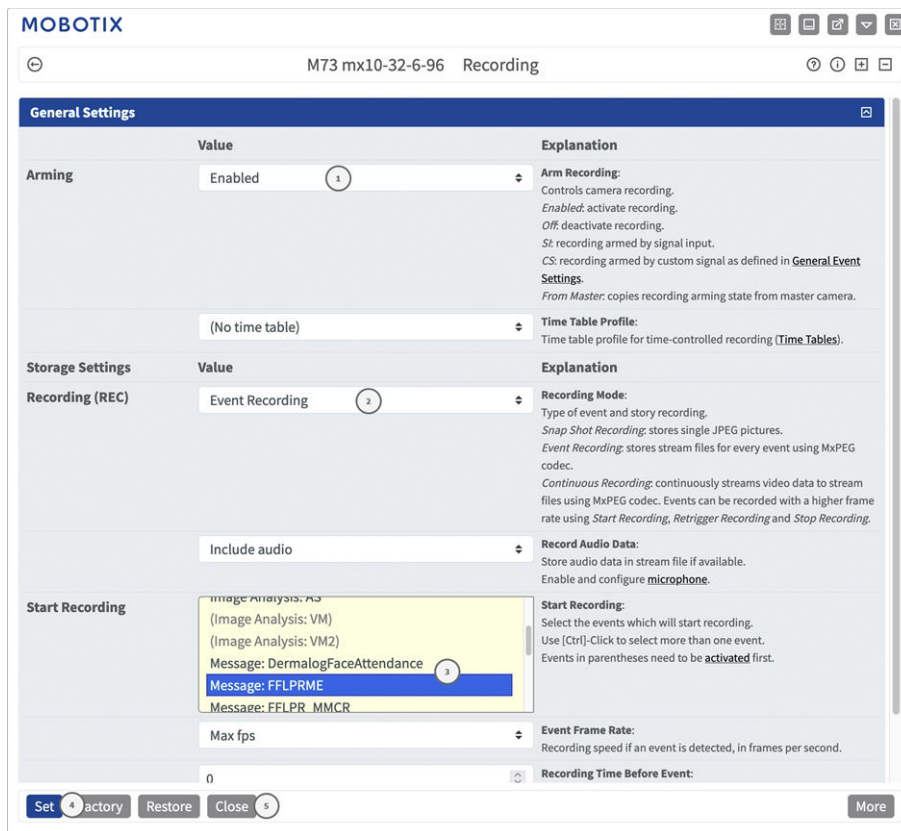
Fig. 34: Configurazione delle impostazioni di registrazione della telecamera
