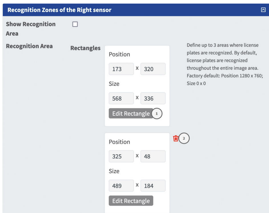
Fig. 22: Scheda "Recognition Areas" (Aree di riconoscimento)
