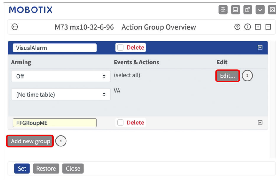
Fig. 31: Definizione dei gruppi di azioni
