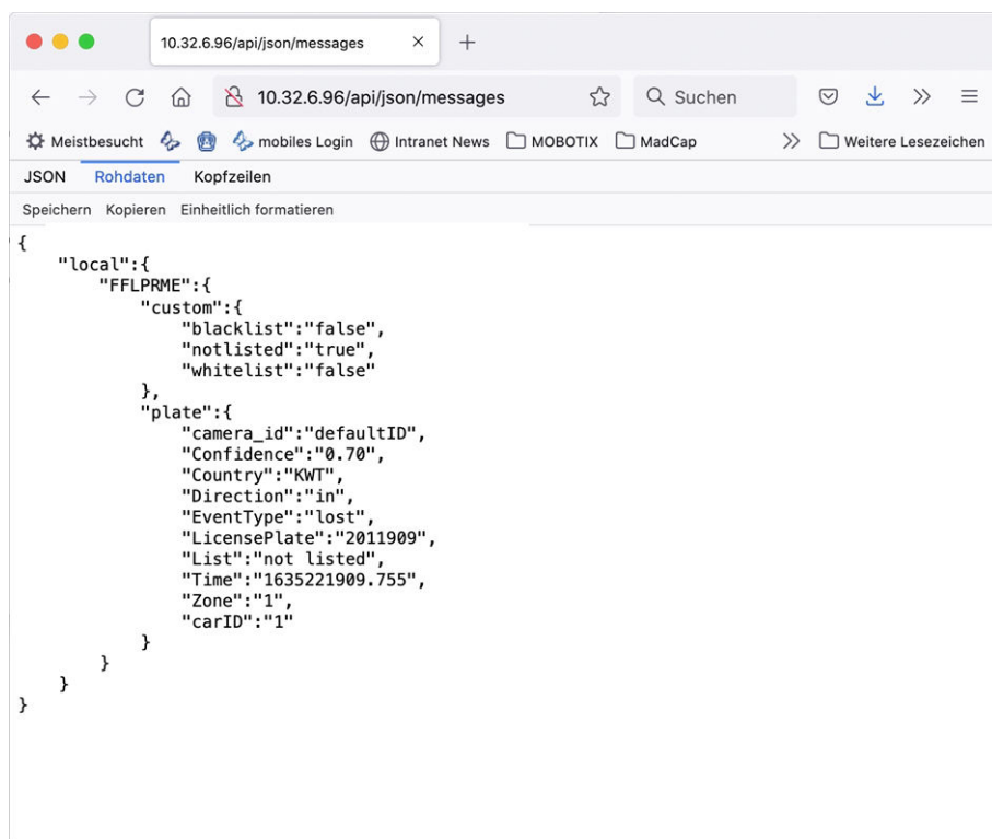
Fig. 35: Esempio: metadati trasmessi all'interno di un MxMessage dell'applicazione FF Group License Plate Recognition App - Region ME
