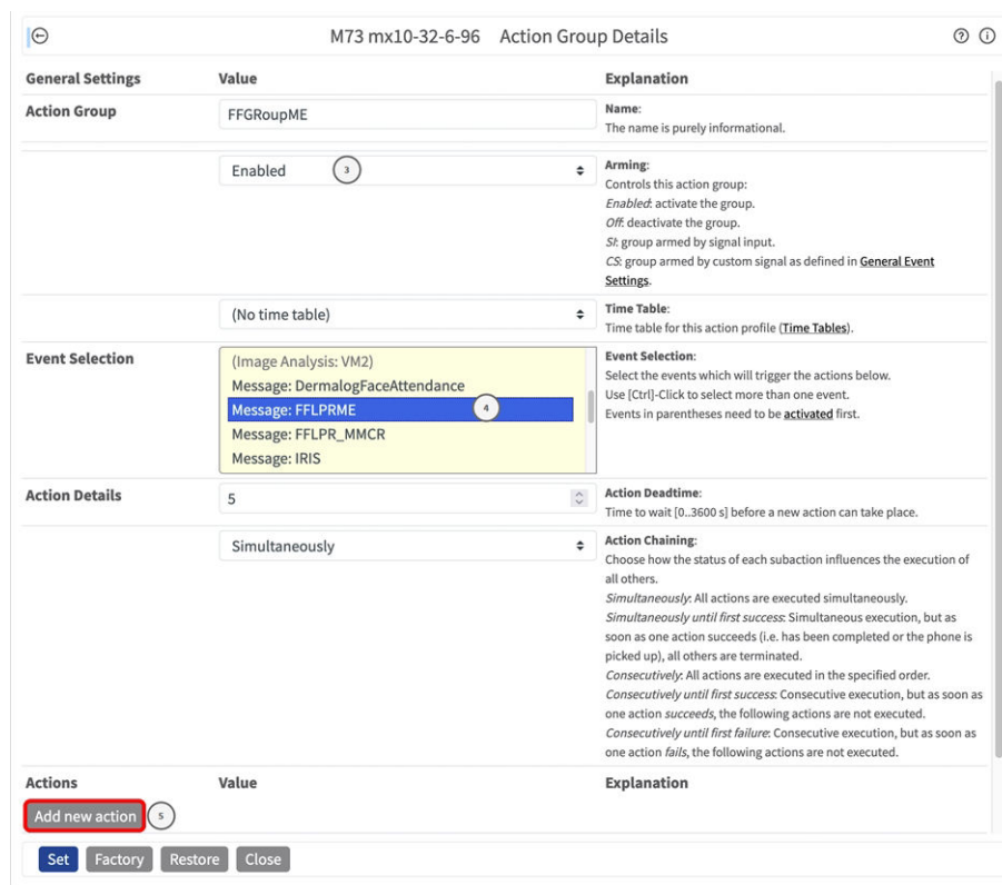
Fig. 32: Configurazione di un gruppo di azioni
