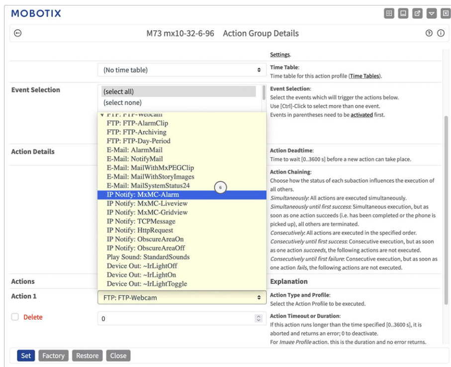
Fig. 33: Selezione del tipo e del profilo dell'azione
