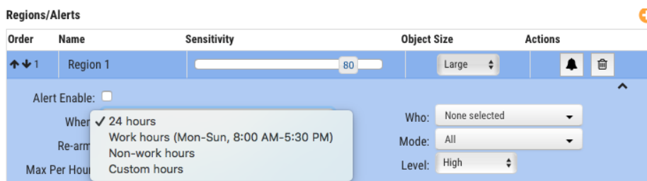
Fig. 66: Alert When
