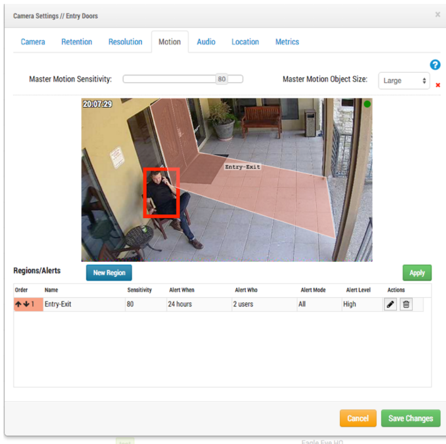
Fig. 69: Alert summary
