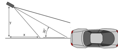
Fig. 13: Allineamento orizzontale della telecamera
