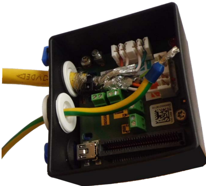
Fig. 61: Filo di massa inserito, tappo posizionato correttamente
