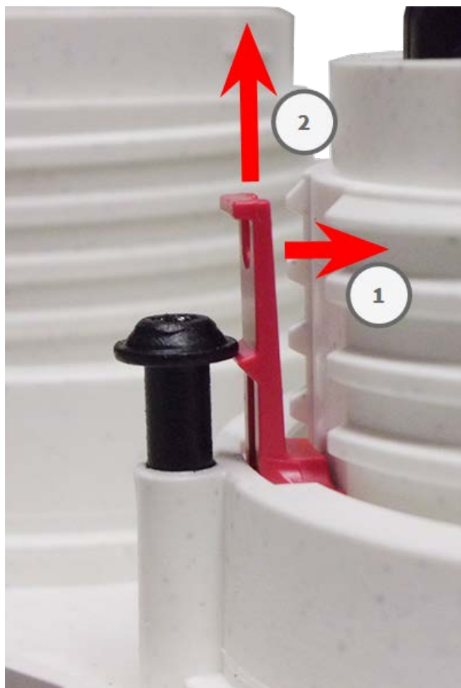
Fig. 19: Rimuovere un fermo di sicurezza
