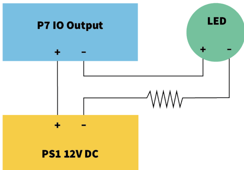
Fig. 67: Esempio: commutazione di un LED
