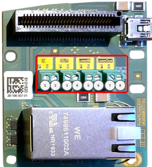
Connettori terminali Connector Box RJ45
