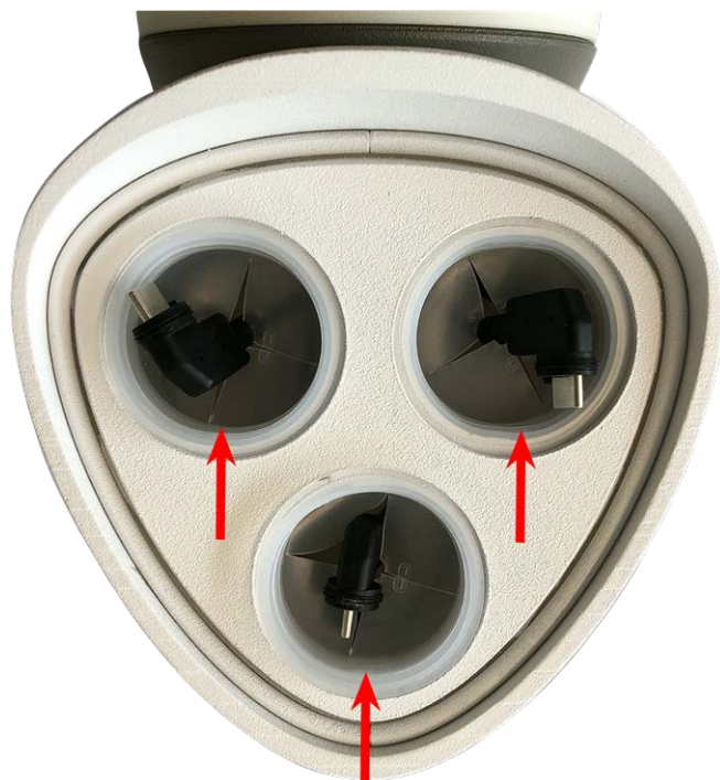
Fig. 7: Rimuovere i tappi di trasporto
