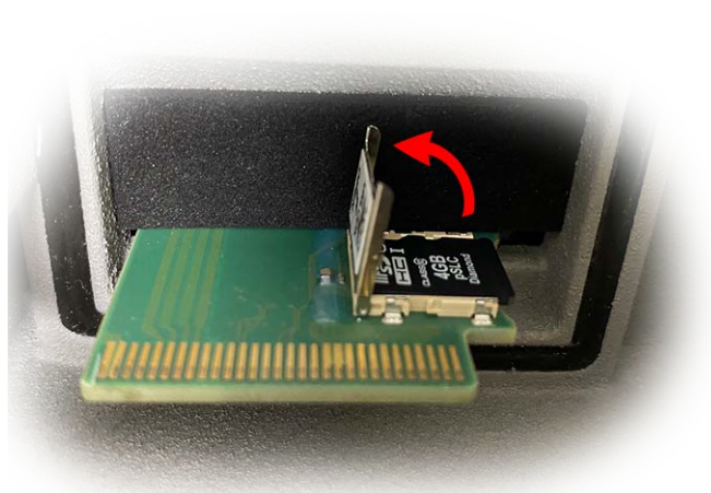
Fig. 95: Sbloccare il supporto della scheda microSD
