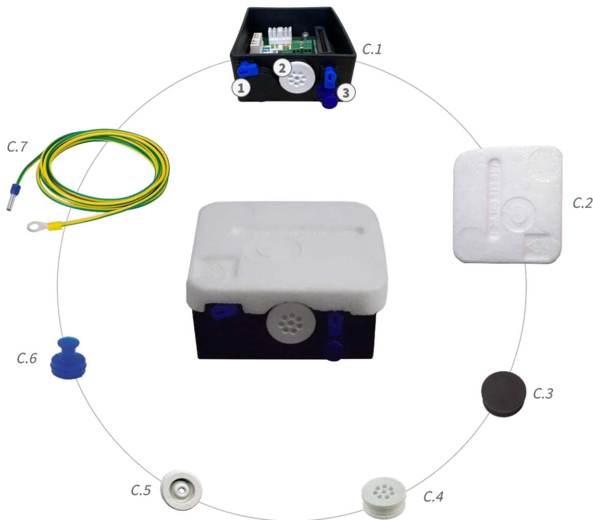
Fig. 3: Contenuto della confezione M73 Connector Box LSA
