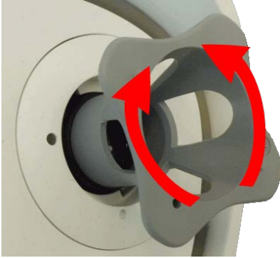
Fig. 84: Regolare la messa a fuoco dell'obiettivo
