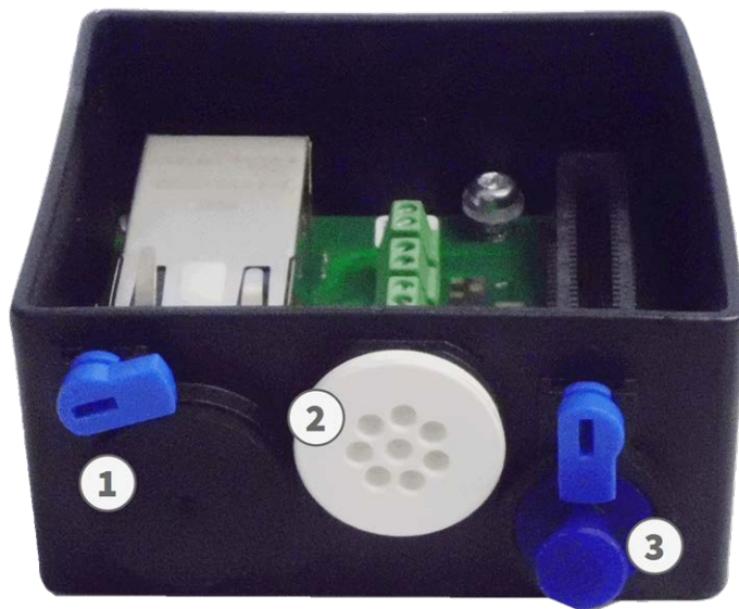
Fig. 64: Connector Box RJ45 con tappo in gomma nero C.3 ① , tappo in gomma a filo singolo C.4 ② , tappo USB ③ e due fermi blu
