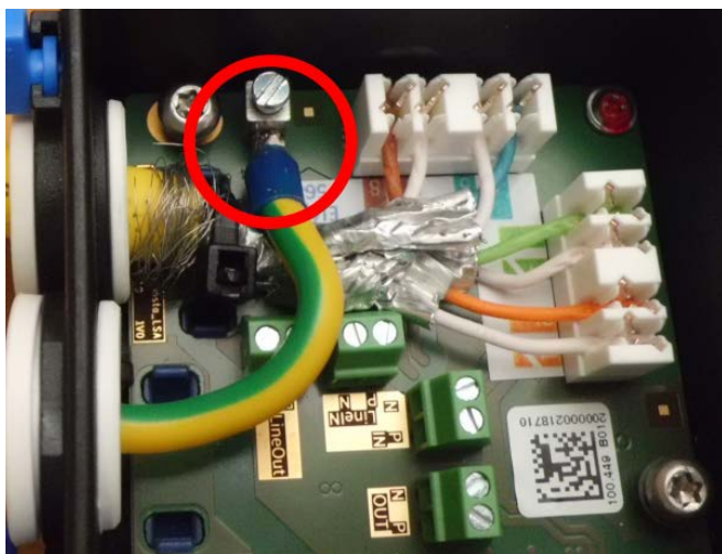
Fig. 62: Filo di massa collegato al morsetto
