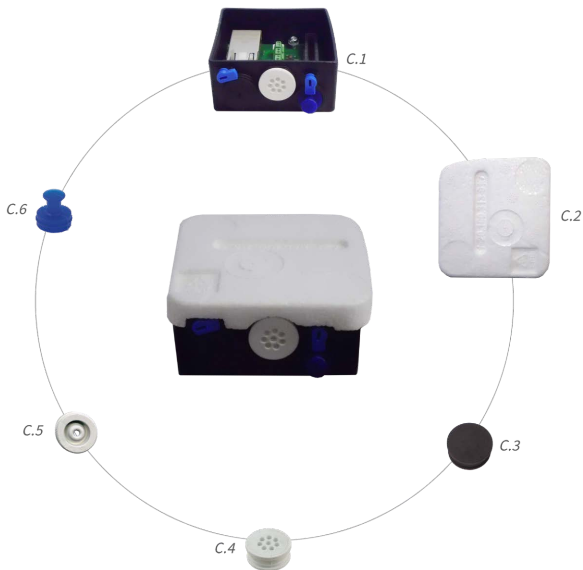
Fig. 2: Contenuto della confezione M73 Connector Box RJ45
