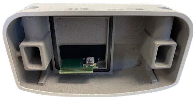
Fig. 94: Aprire il corpo della telecamera
