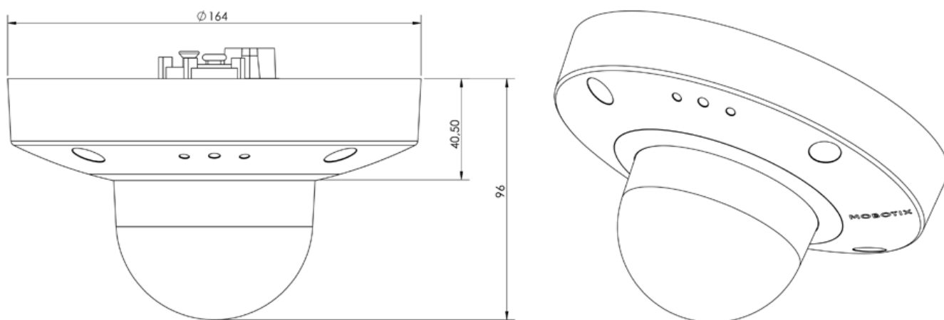
Abb. 1: D71: Alle Maßangaben in mm
