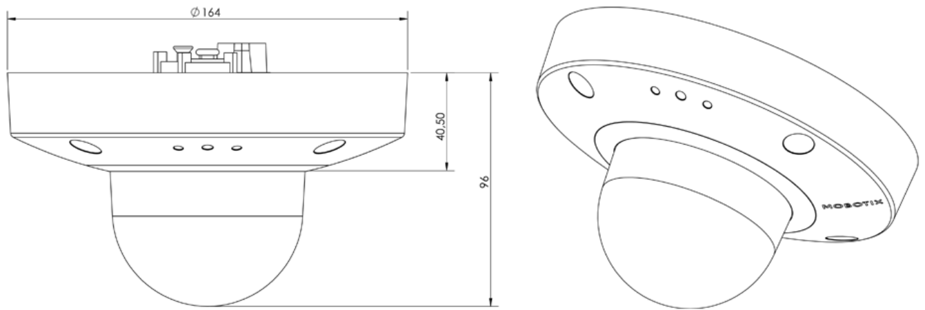
Fig. 1: D71: Todas las medidas en mm
