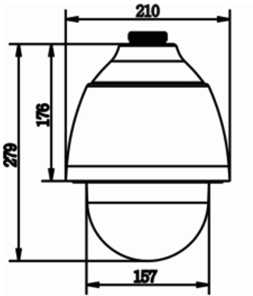
図1: MOBOTIX MOVE SpeedDome: すべての測定値の単位はmm
