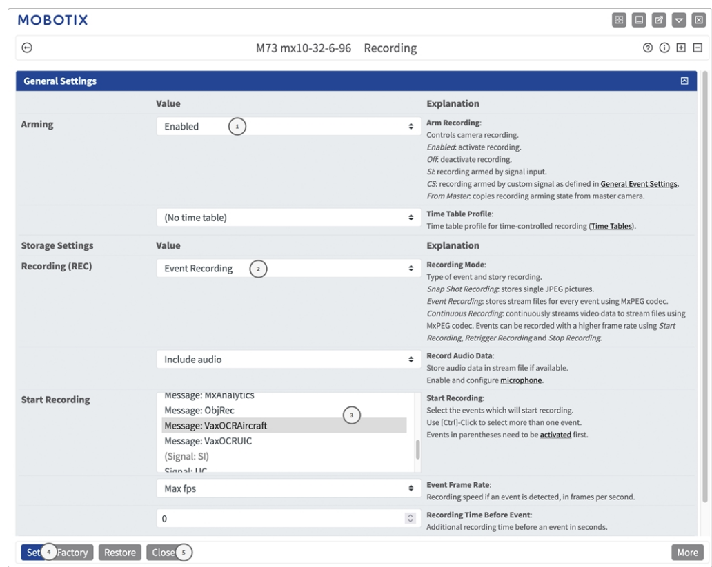
Fig. 28: Configuración de los ajustes de grabación de la cámara
