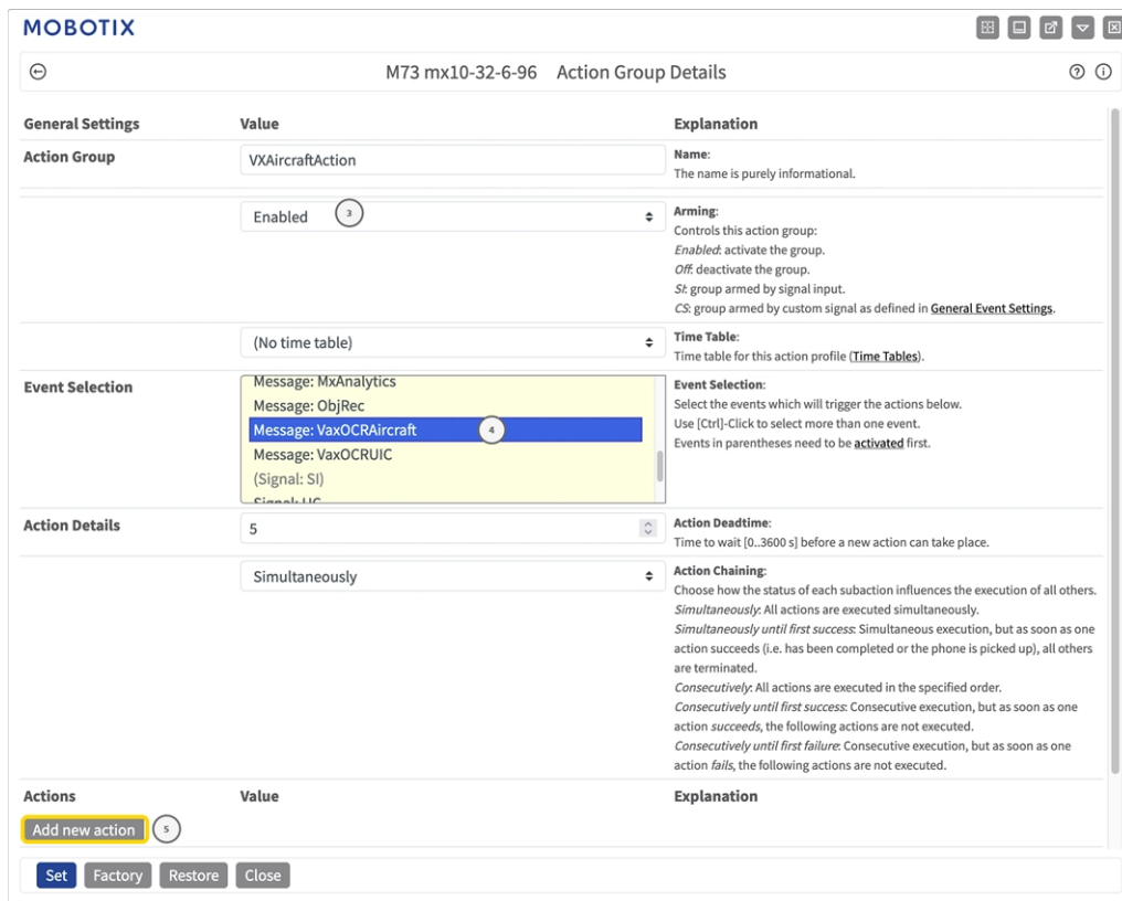
Fig. 26: Configuración de un grupo de acciones
