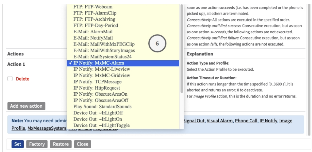
Fig. 27: Selección de tipo de acción y perfil
