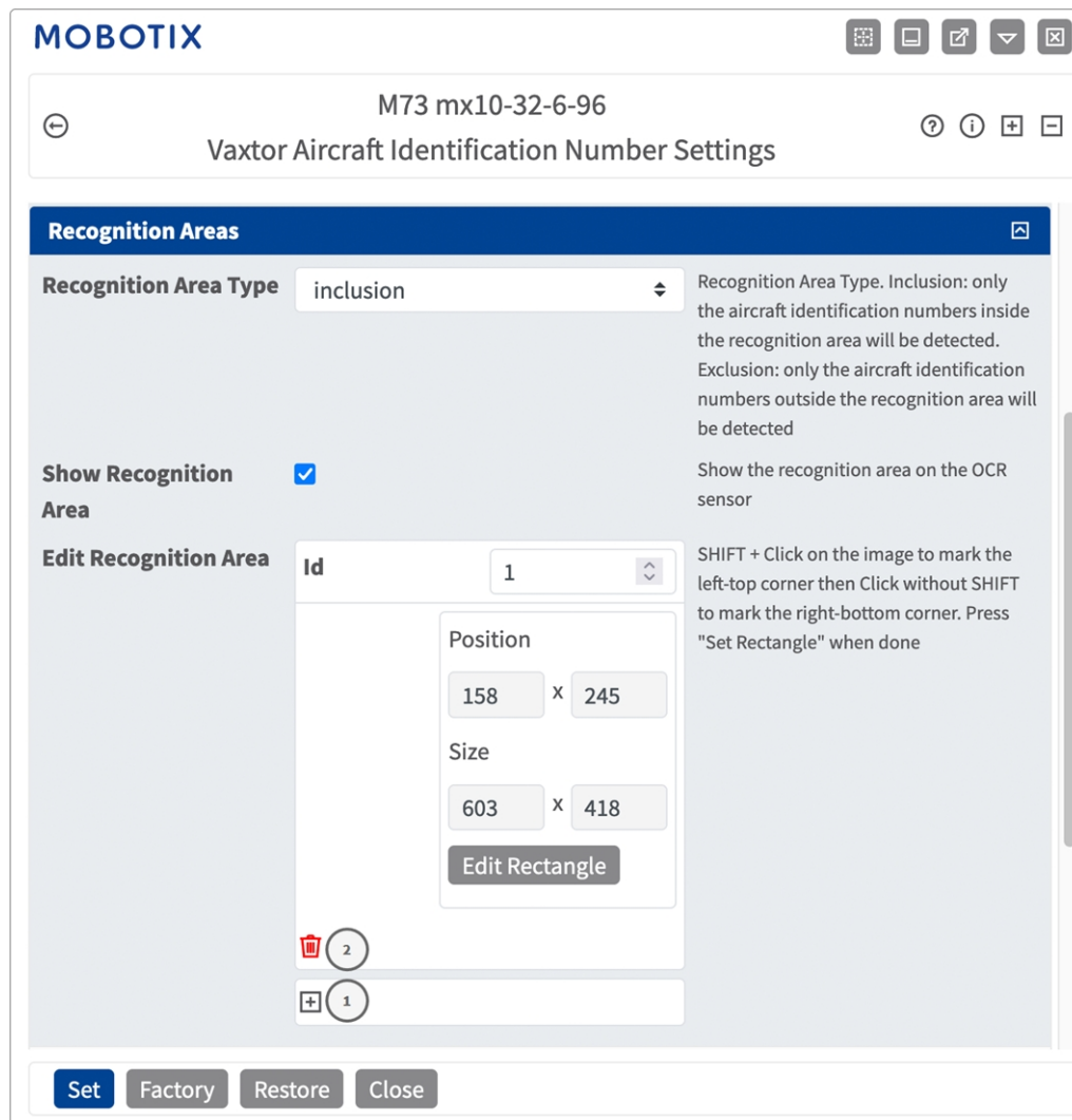
Fig. 14: Áreas de reconocimiento
