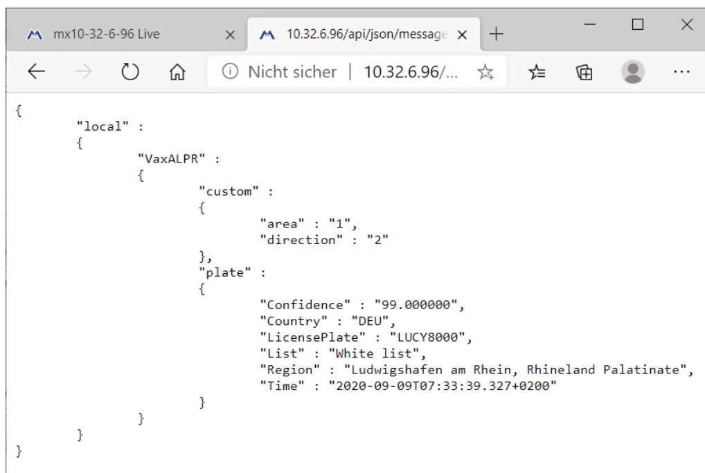
Abb. 29: Beispiel: Metadaten, die innerhalb einer MxMessage von Vaxtor License Plate Recognition App übertragen werden
