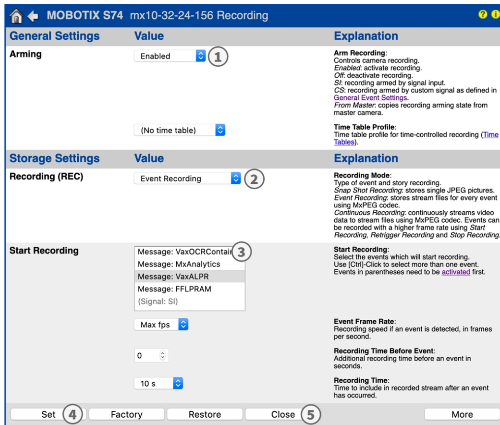
Abb. 28: Konfiguration der Aufnahmeeinstellungen der Kamera
