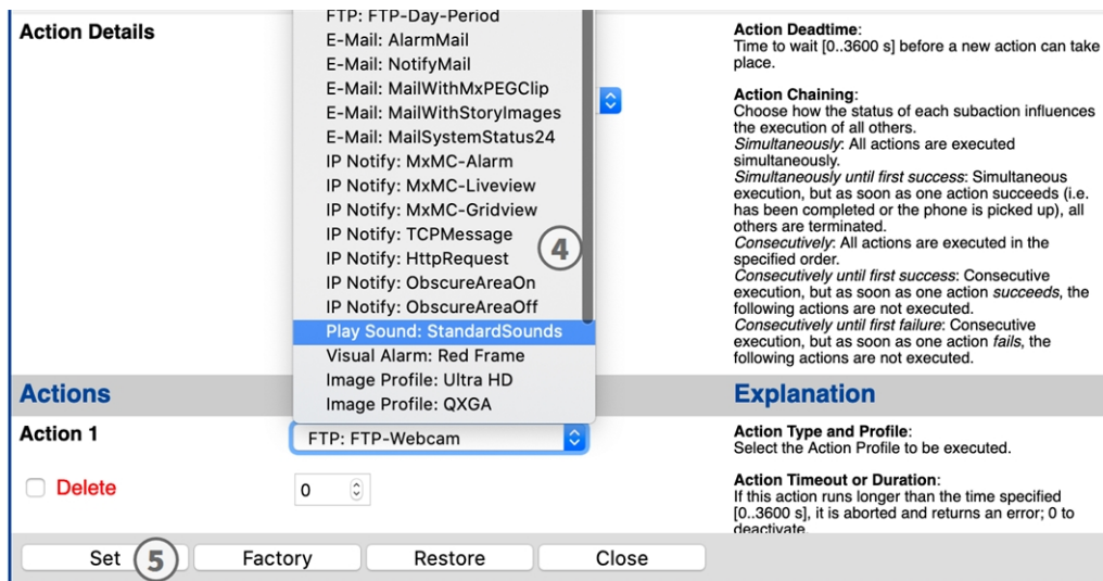
Abb. 27: Aktionstyp und Profil auswählen
