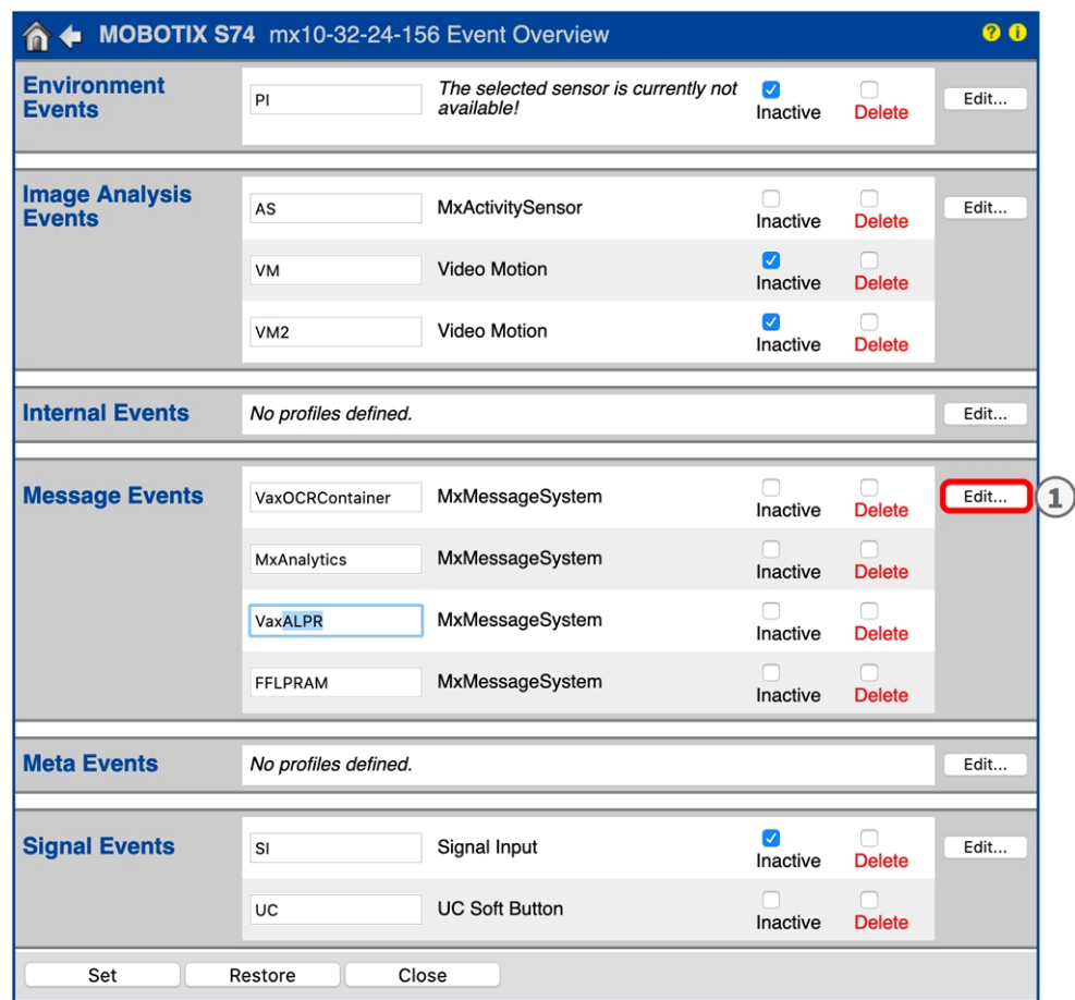
Fig. 23: Esempio: evento messaggio generico da Vaxtor License Plate Recognition App
