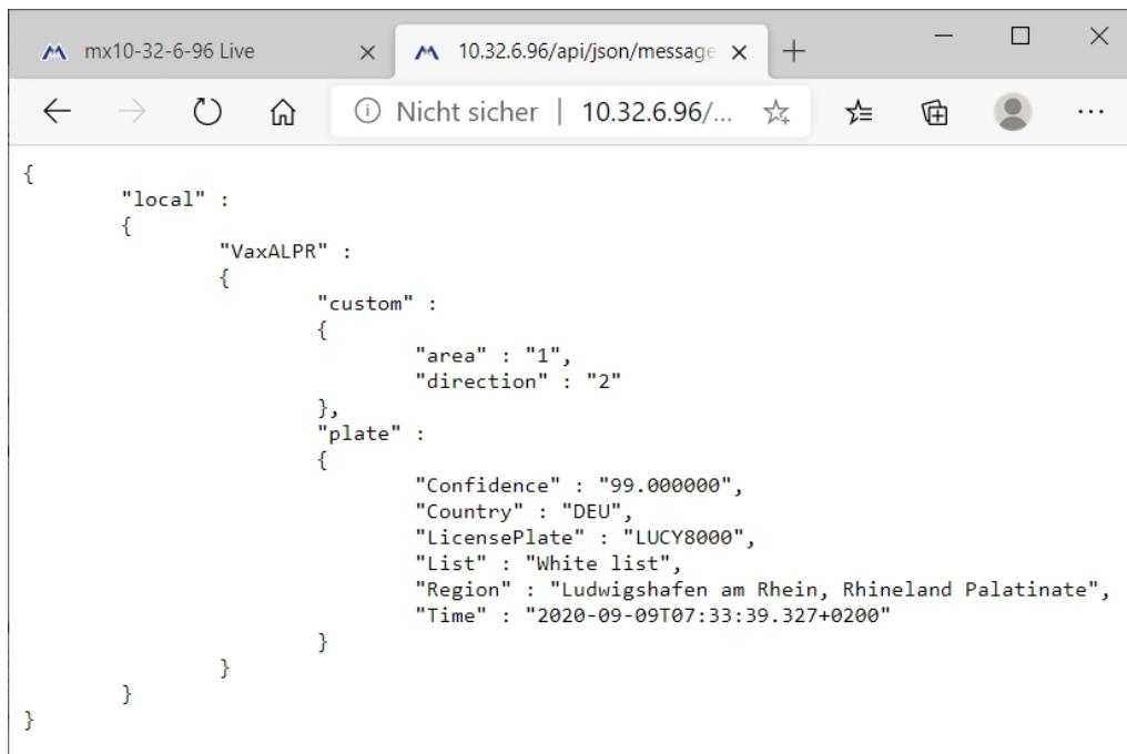
Fig. 29: Esempio: metadati trasmessi all'interno di un MxMessage dell'applicazione Vaxtor License Plate Recognition App
