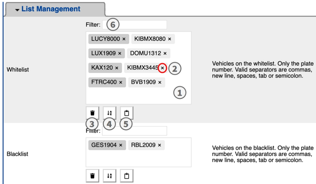
Fig. 15: Lista bianca e lista nera
