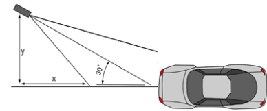
Fig. 13: Alineación horizontal de la cámara
