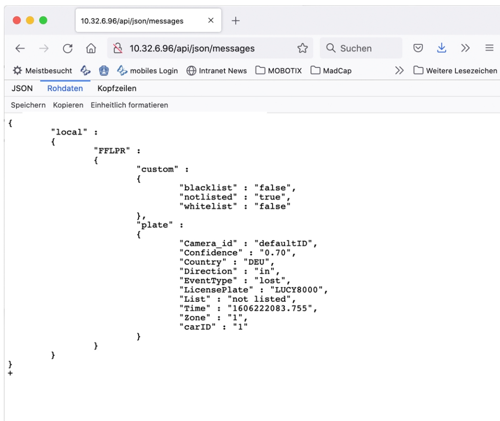
Fig. 35: Ejemplo: Metadatos transmitidos dentro de un MxMessage de FF Group License Plate Recognition App - Region EUCA
