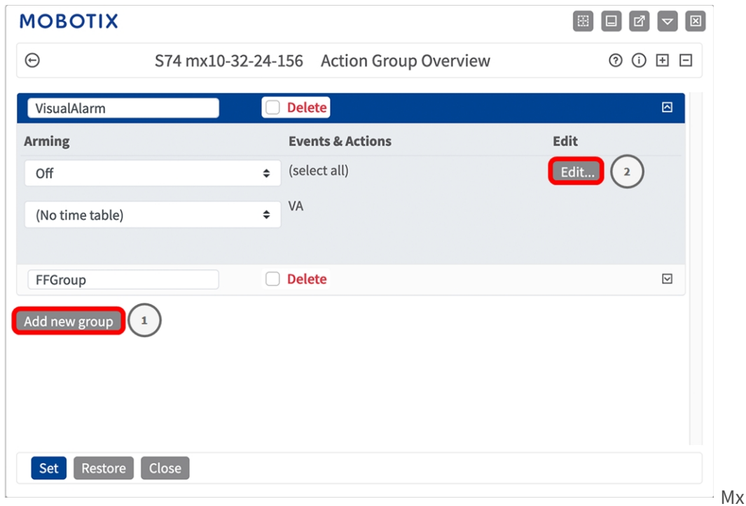
Fig. 31: Définir des groupes d'actions
