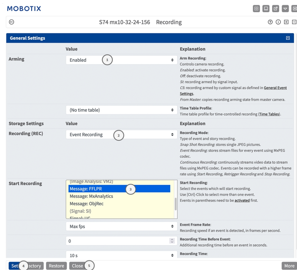
Fig. 34: Configuration des paramètres d'enregistrement de la caméra
