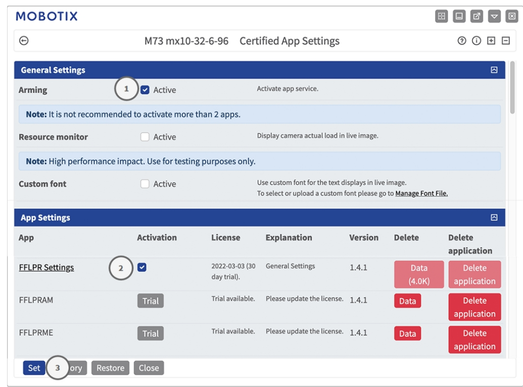
Fig. 20: App certifiée : Configuration
