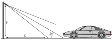
Fig. 10: Pointage vertical de la caméra
