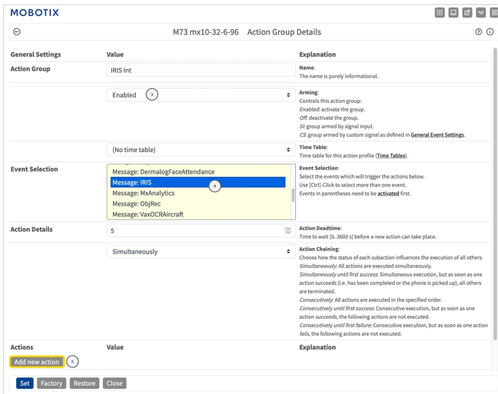
Fig. 22: Configurazione di un gruppo di azioni
