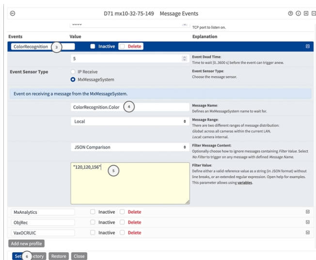
Abb. 20: Beispiel: Schwarze-Liste-Nachrichtenereignis
