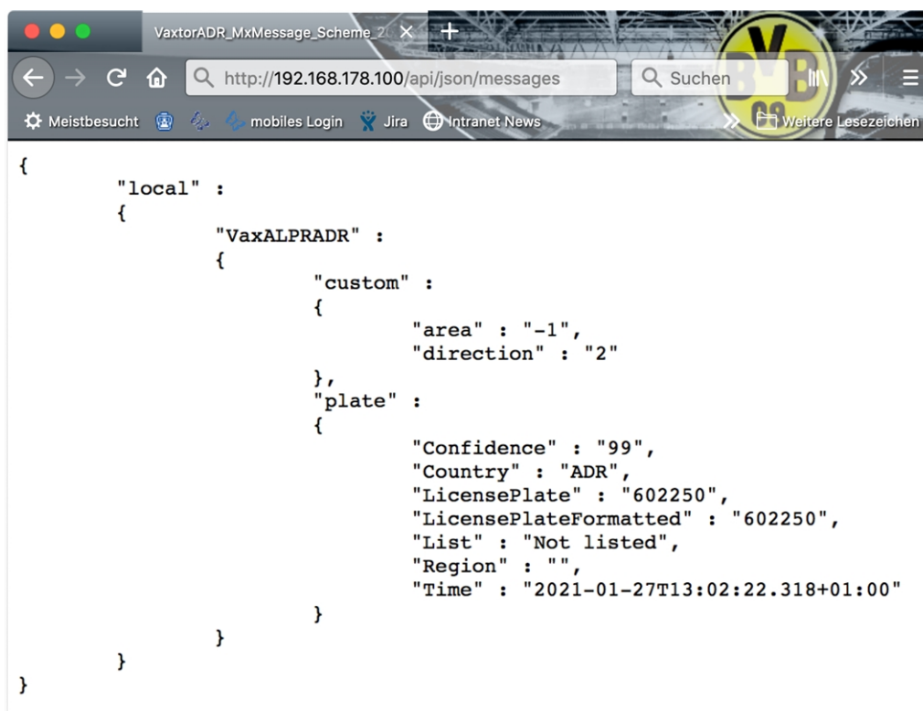
Abb. 27: Beispiel: Metadaten, die innerhalb einer MxMessage von Vaxtor License Plate Recognition / Dangerous Goods App übertragen werden
