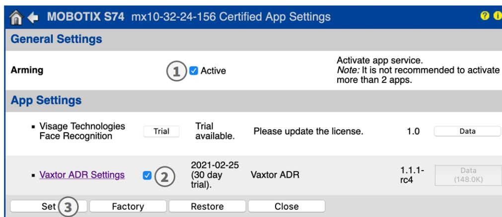
Abb. 12: Aktivierung zertifizierter Apps
