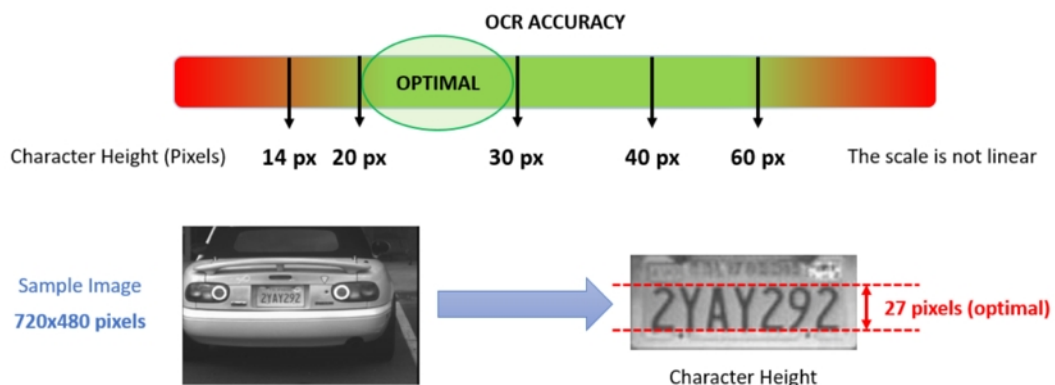
Abb. 10: Minimale Zeichenhöhe
