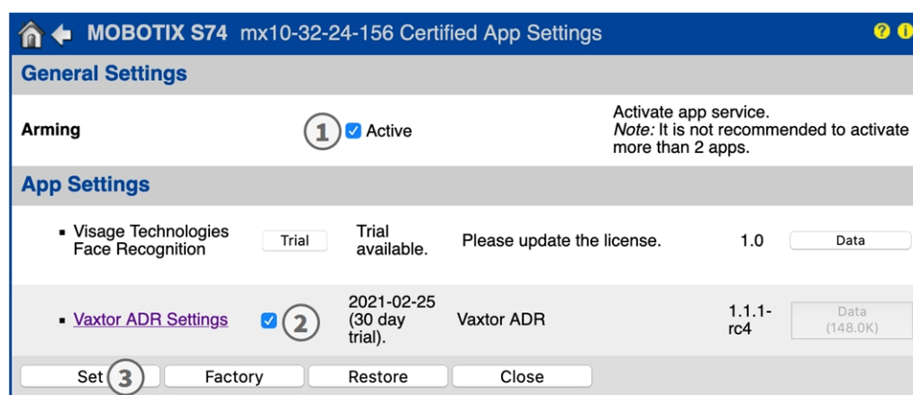
Fig. 12: Attivazione delle applicazione certificate
