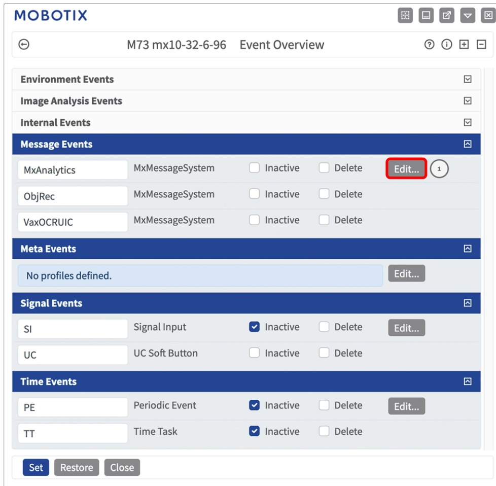
Abb. 31: Beispiel: Generisches Nachrichtenereignis von Vaxtor Aircraft Identification Number Recognition App
