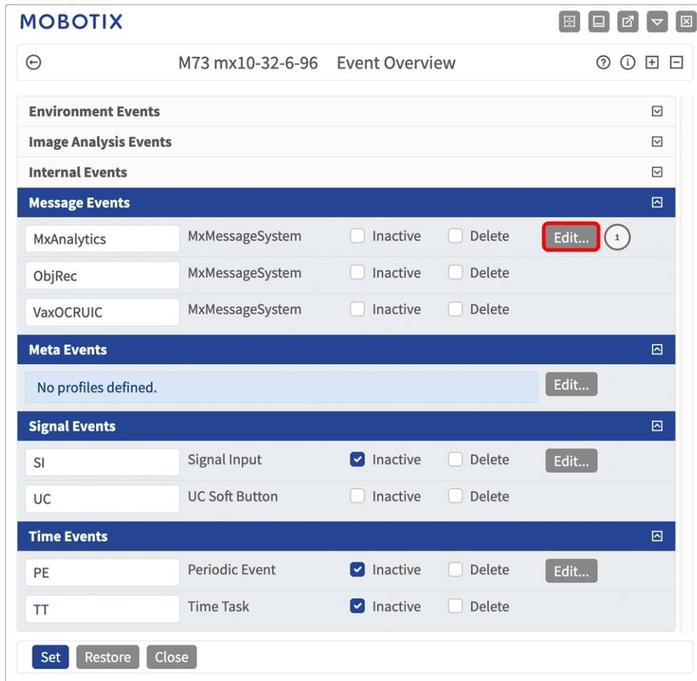
Fig. 31: Esempio: Evento messaggio generico da Vaxtor Aircraft Identification Number Recognition App
