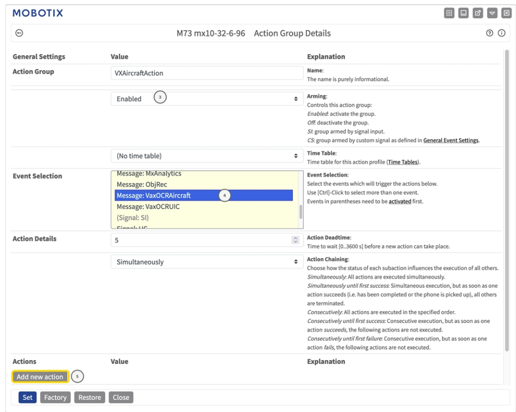
Fig. 26: Configurazione di un gruppo di azioni
