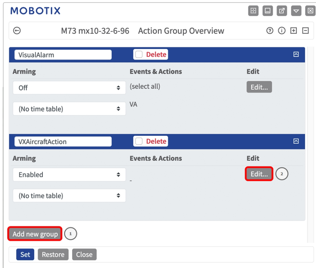
Fig. 25: Definizione dei gruppi di azioni
