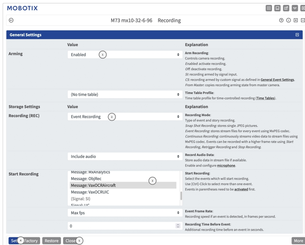
Fig. 28: Configurazione delle impostazioni di registrazione della telecamera
