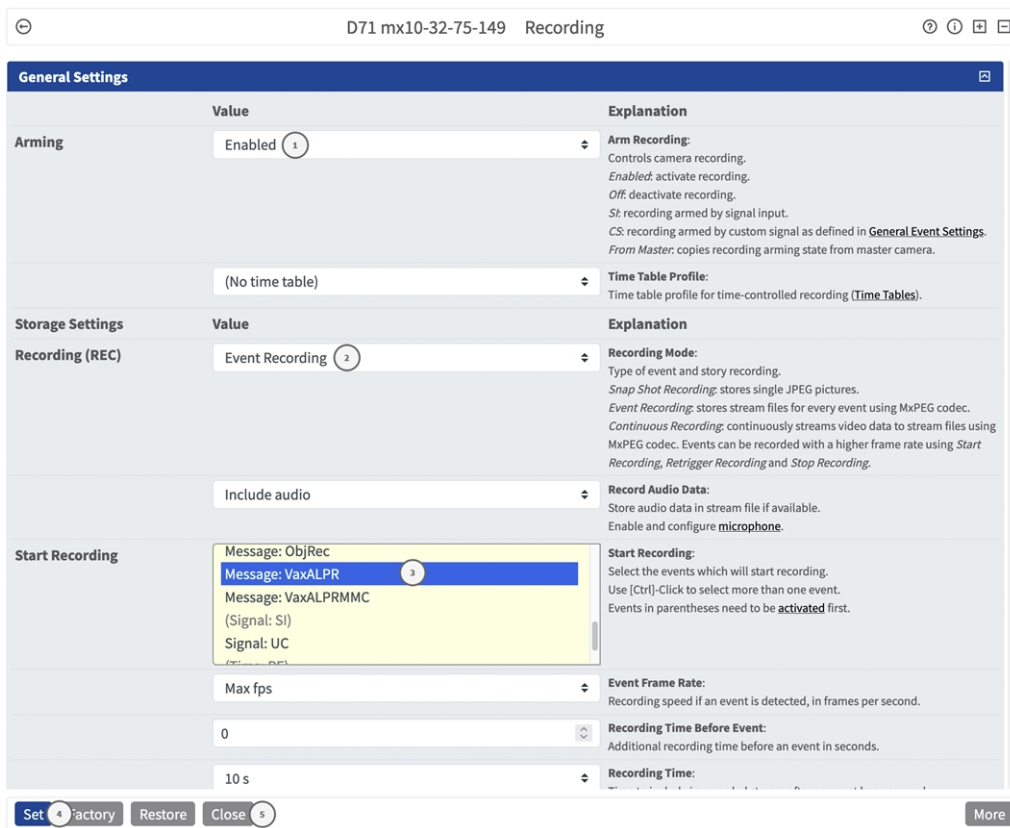
Fig. 25: Configurazione delle impostazioni di registrazione della telecamera
