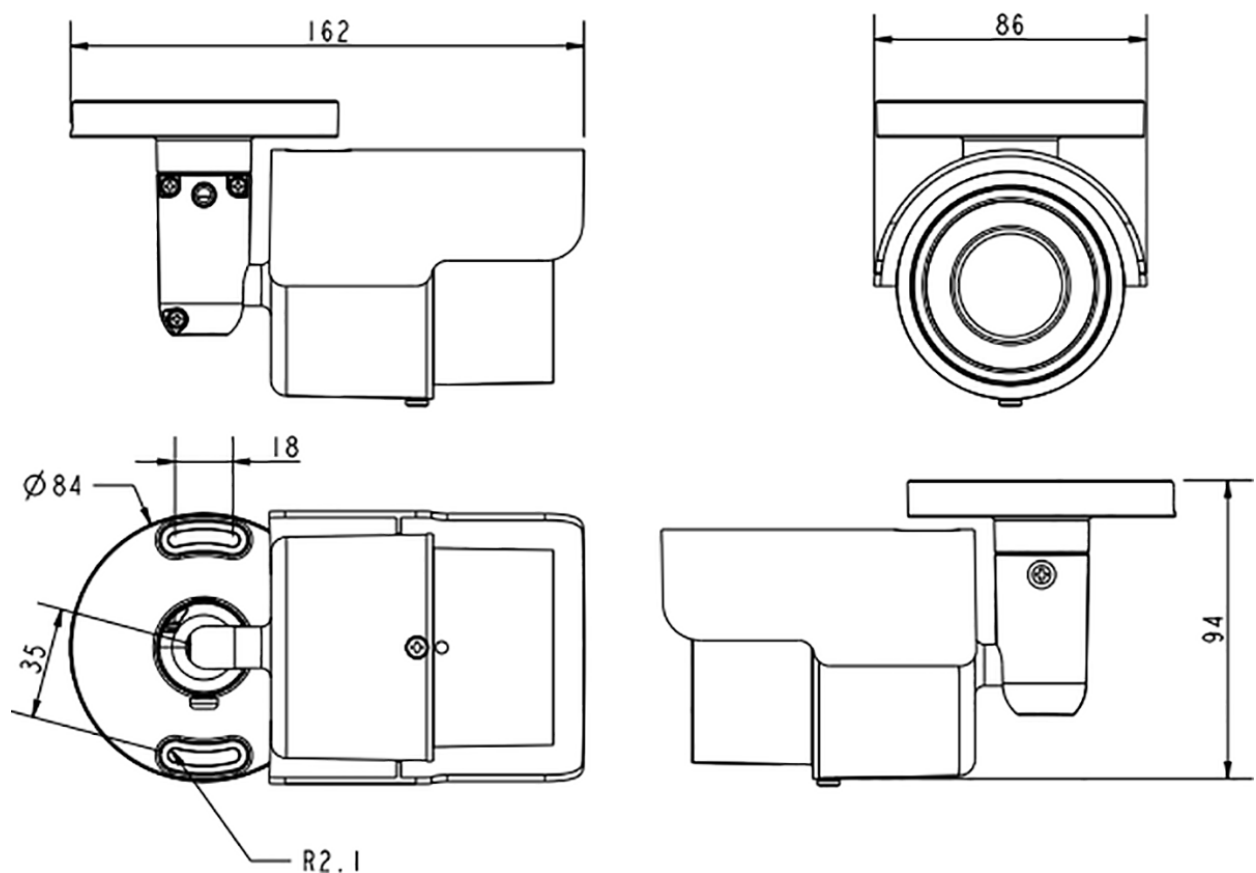
Abb. 1: 2MP Bullet Camera: Alle Maßangaben in mm
