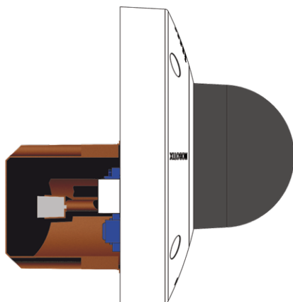
Abb. 6: Seitenansicht der MOBOTIX D71 über Unterputzsteckdose
