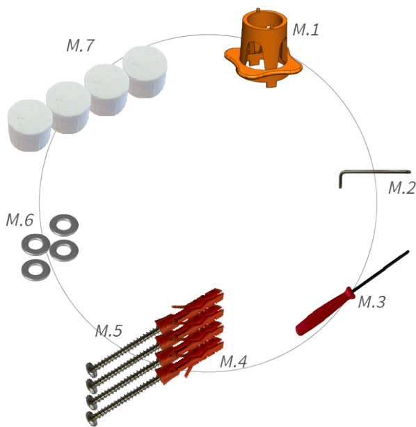
Abb. 2: Lieferumfang MOBOTIX D71 Montagezubehör
