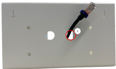
Abb. 15: Netzwerkverkabelung vorbereiten
