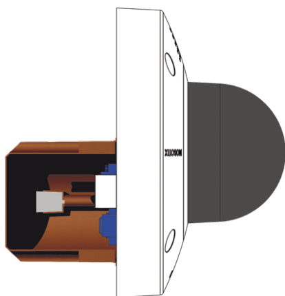
Fig. 6: Vue latérale de la MOBOTIX D71 sur prise murale encastrée
