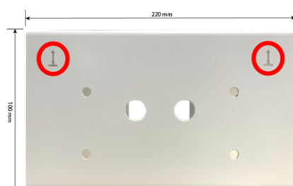
Fig. 10: Dimensions MOBOTIX D71 Corner/Pole Mount – vue avant
