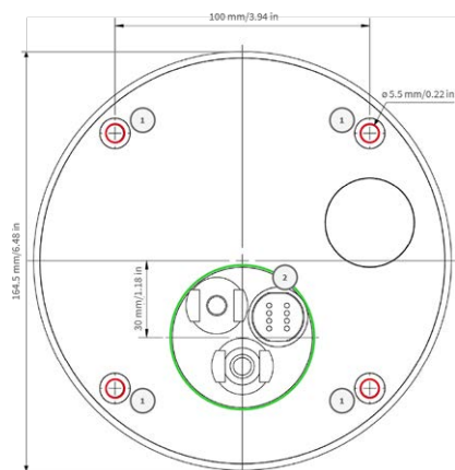
Fig. 7: Gabarit de perçage avec trous pour le positionnement des vis de fixation (cercles rouges) et pour la prise murale encastrée (cercle vert)
