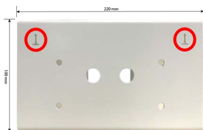
Fig. 10: Dimensions MOBOTIX Q71 Corner/Pole Mount – vue avant
