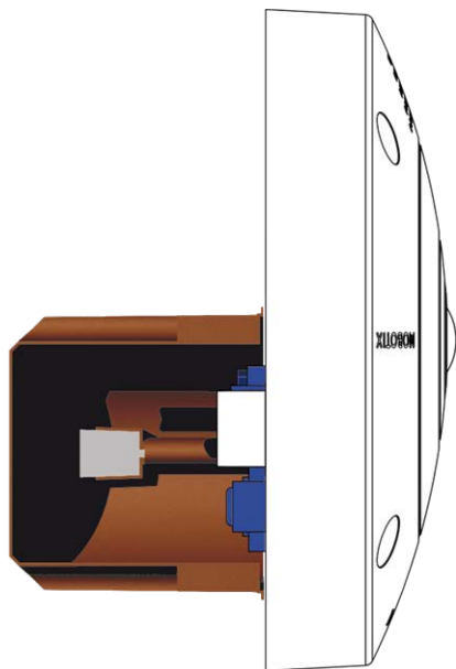
Fig. 6: Vue latérale de la MOBOTIX Q71 sur prise murale encastrée
