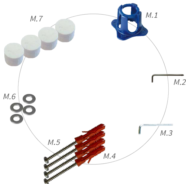
Fig. 2: Contenu de la livraison : accessoires de montage de MOBOTIX Q71
