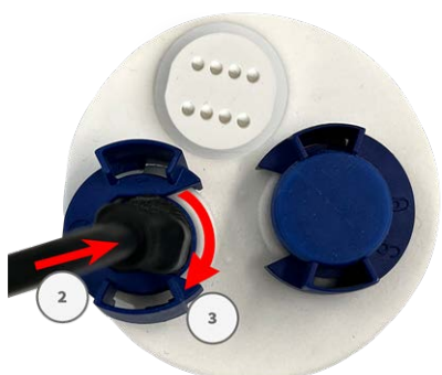
Fig. 16: Appuyez fermement sur la fiche jusqu'à ce que la bague d'étanchéité bleue s'enclenche
