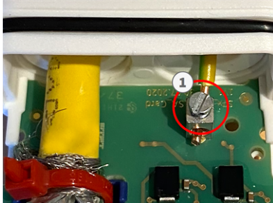
Fig. 28: Cable de tierra conectado al borne
