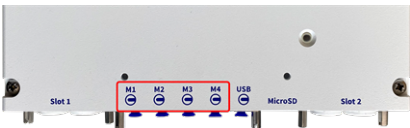
Fig. 39: Conectores del módulo de MOBOTIX S74
