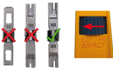
Fig. 25: Herramienta LSA+/Krone ajustada a un impacto BAJO
