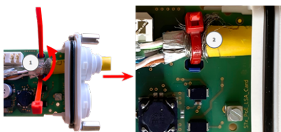
Fig. 24: Brida introducida debajo del cable de red
