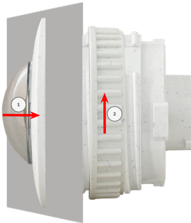
Fig. 10: Monte el módulo del sensor
