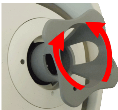
Fig. 53: Ajuste el enfoque del objetivo
