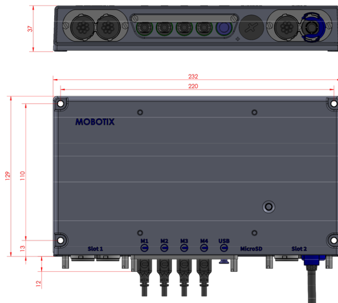
Fig. 5: MOBOTIX S74: Todas las medidas en mm
