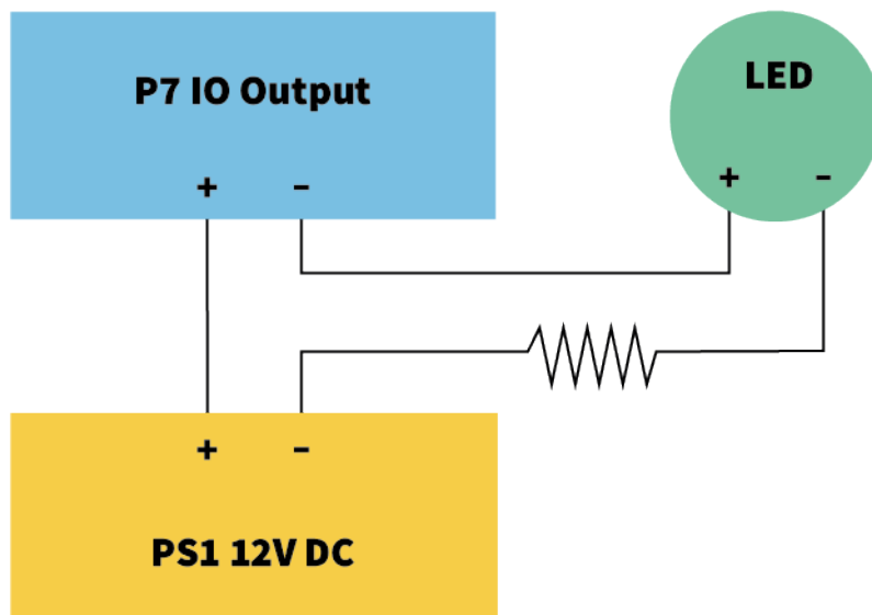
Fig. 35: Ejemplo: encendido de un LED
