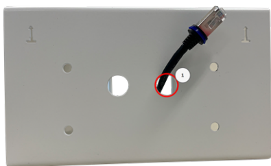
Abb. 12: Netzwerkverkabelung vorbereiten
