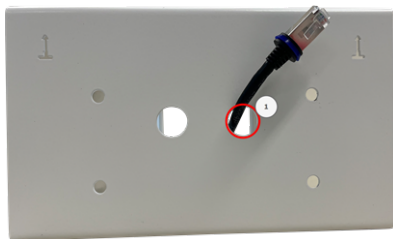
Abb. 15: Netzwerkverkabelung vorbereiten
