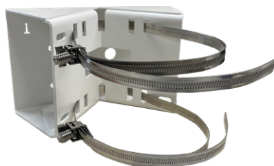
Fig. 13: Préparez le support sur poteau avec des sangles en acier
