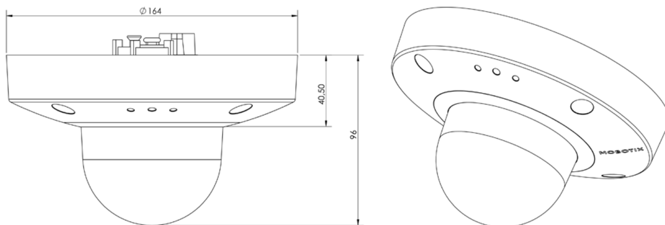
Fig. 5: MOBOTIX v71: Todas las medidas en mm
