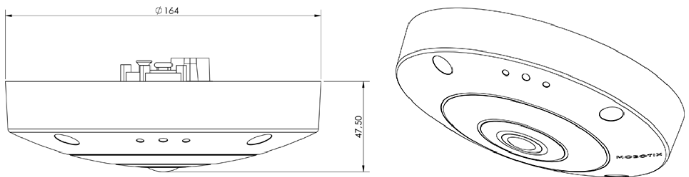
Fig. 1: MOBOTIX Q71 : toutes les mesures sont en mm
