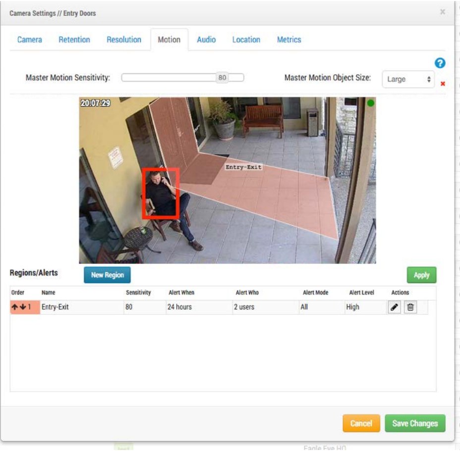
Fig. 71: Alert summary
