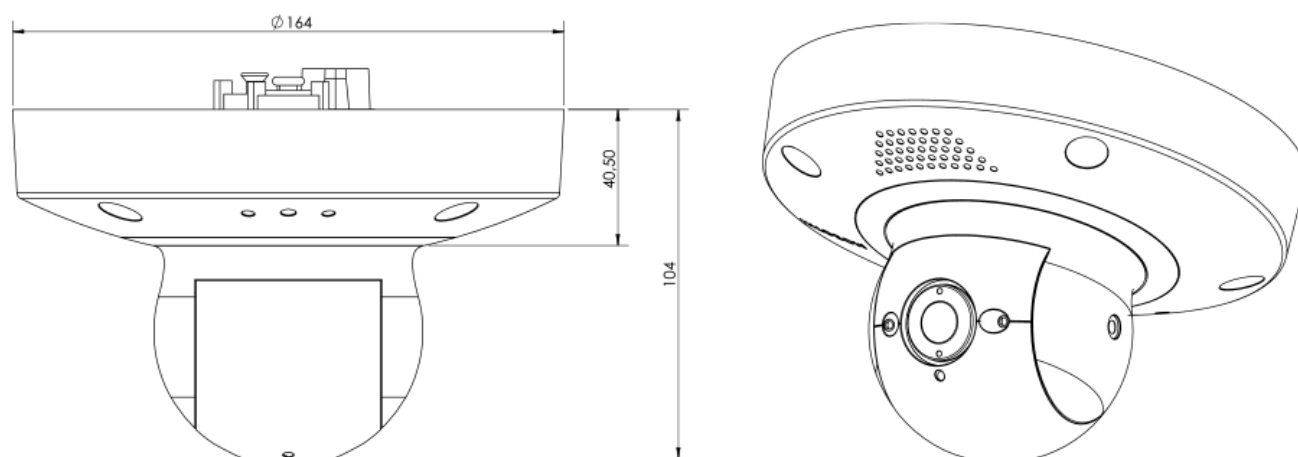
Fig. 5: MOBOTIX p71: Todas las medidas en mm
