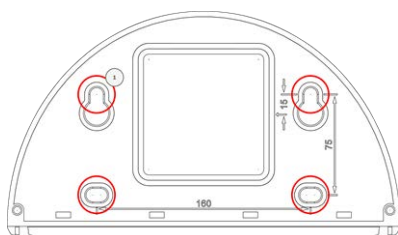
Fig. 8: Wall Mount avec trous pour le positionnement des vis de fixation
