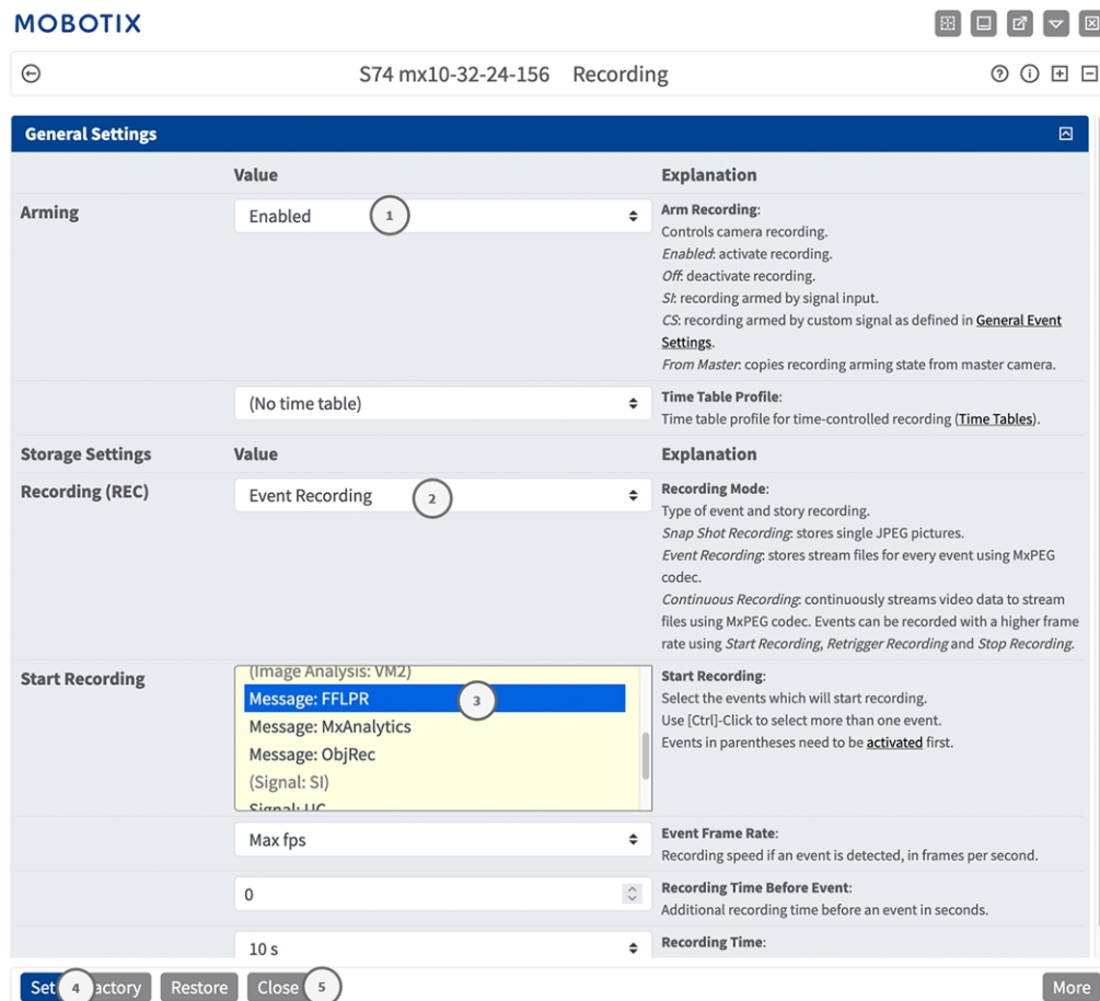
Fig. 34: Configurazione delle impostazioni di registrazione della telecamera
