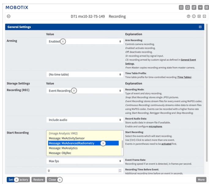
Fig. 20: Configurazione delle impostazioni di registrazione della telecamera
