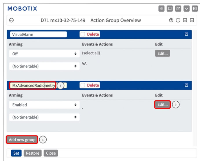
Fig. 17: Definizione dei gruppi di azioni
