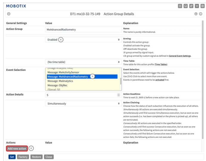
Fig. 18: Configurazione di un gruppo di azioni
