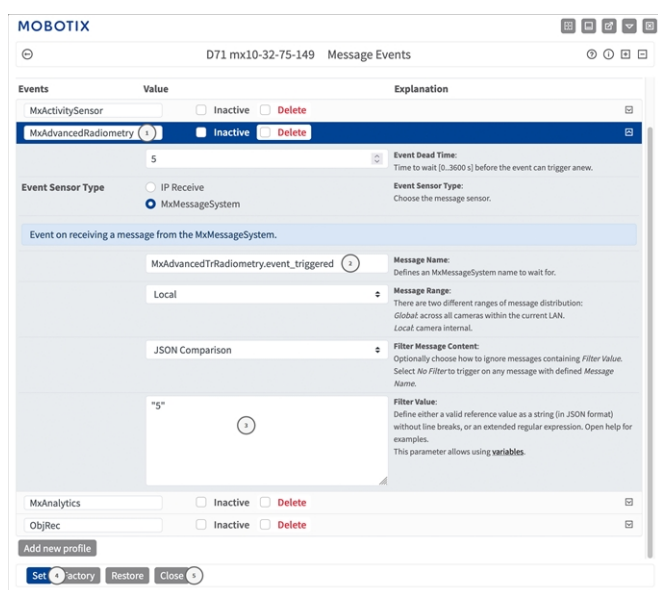
Fig. 23: Esempio: Evento targa univoca
