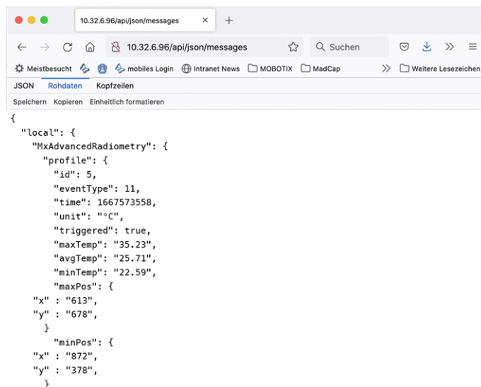
Fig. 21: Esempio: metadati trasmessi all'interno di un MxMessage di MOBOTIX Advanced Radiometry App
