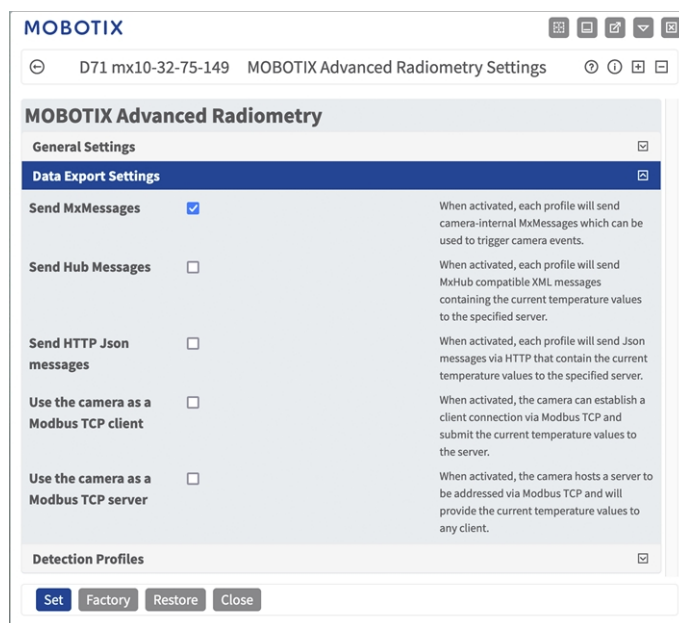
Fig. 12: Impostazione di esportazione dei dati
