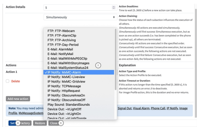
Fig. 19: Selezione del tipo e del profilo dell'azione
