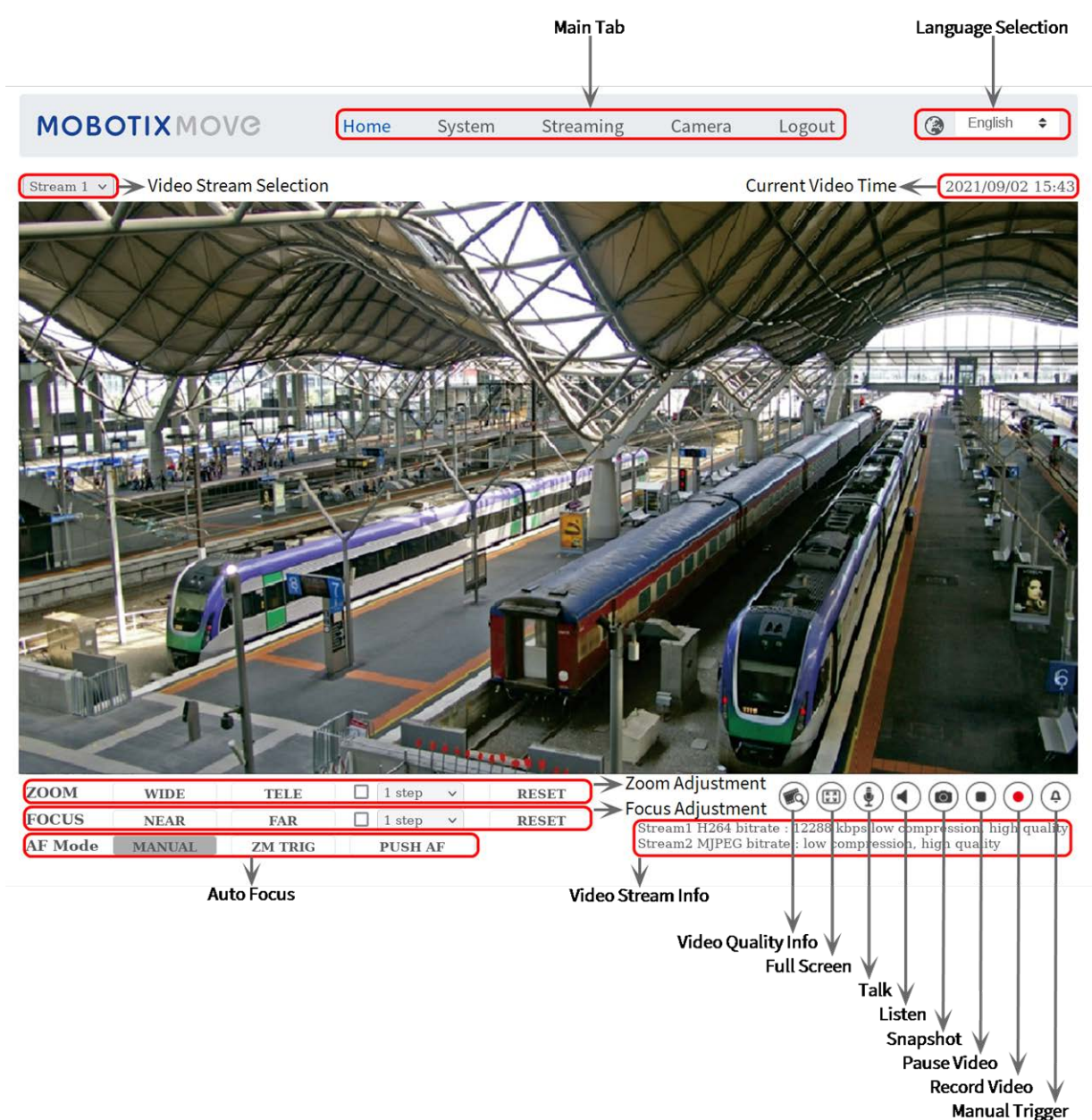
Fig. 2: Fenêtre de visualisation
