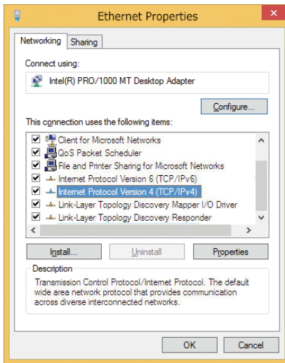
Abb. 76: Netzwerkeinstellungen auf Windows-Computern
