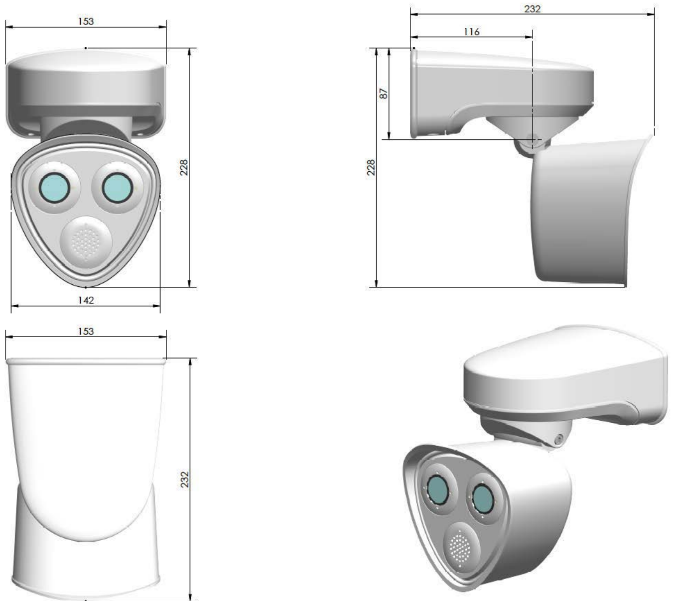
Abb. 5: MOBOTIX M73: Alle Maßangaben in mm
