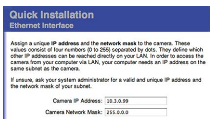
Abb. 79: Netzwerkeinstellungen in der Weboberfläche der Kamera
