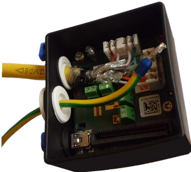
Abb. 62: Masseleitung eingesteckt, Stopfen richtig eingesetzt
