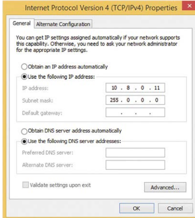
Abb. 77: Eigenschaften von Internet Protocol V4
