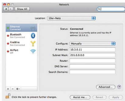
Abb. 78: Netzwerkeinstellungen auf macOS-Computern
