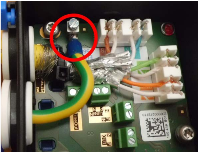
Abb. 63: Masseleitung mit Klemme verbunden
