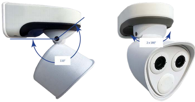
Abb. 30: Neigbarkeit bei Wandmontage
