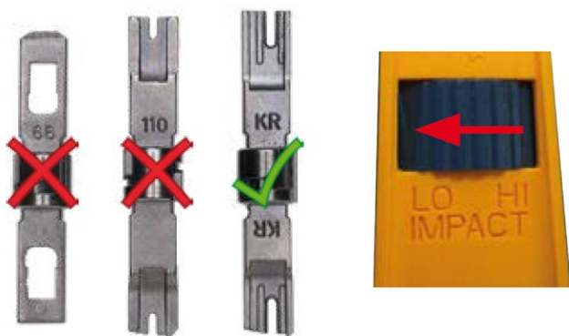
Abb. 59: Krone LSA-Plus-Anlegewerkzeug auf GERINGE Kraft eingestellt
