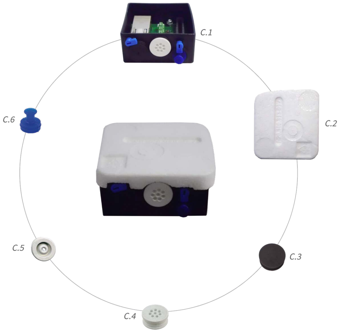
Abb. 2: Lieferumfang MOBOTIX M73 Connector Box RJ45
