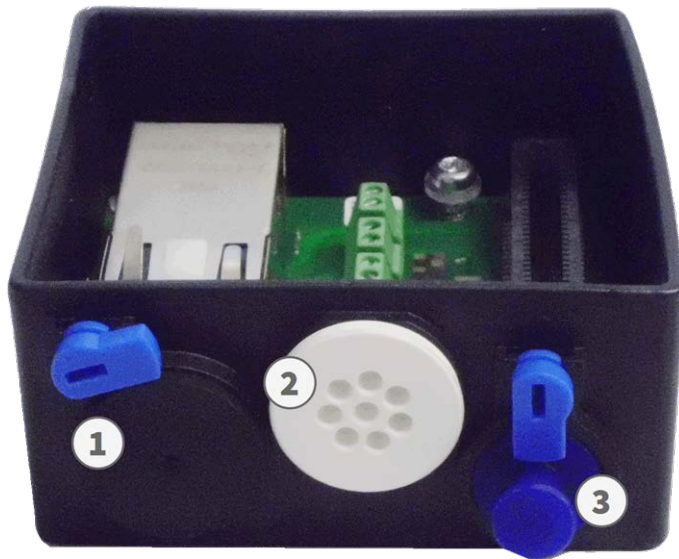
Abb. 65: Connector Box RJ45 mit Gummistopfen, schwarz C.3 ① ; Gummistopfen, einadrig C.4 ② ; USB-Stecker ① und zwei blauen Verriegelungen
