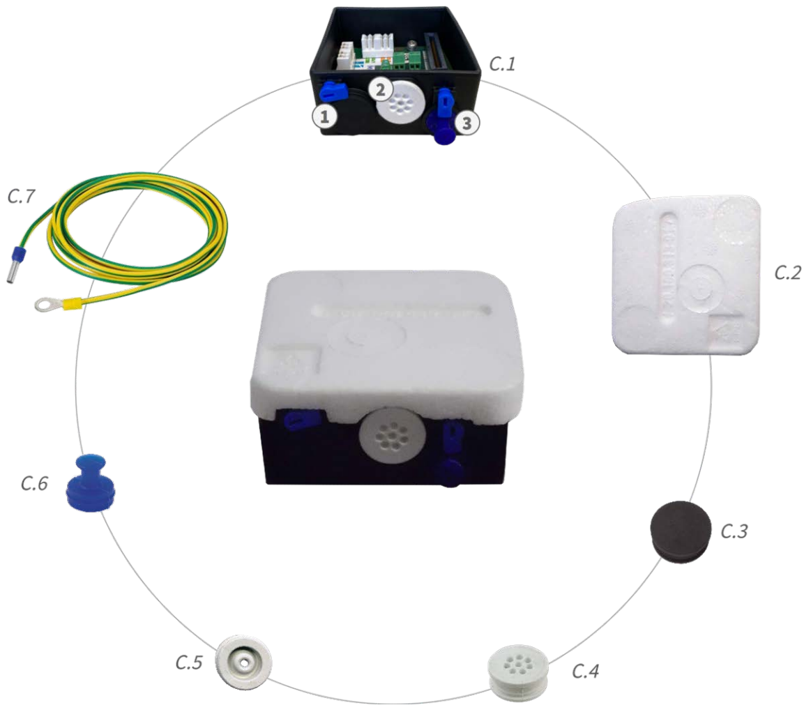
Abb. 3: Lieferumfang MOBOTIX M73 Connector Box LSA
