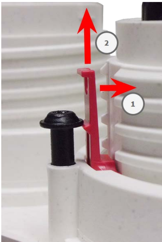
Abb. 20: Sicherungsclip entfernen
