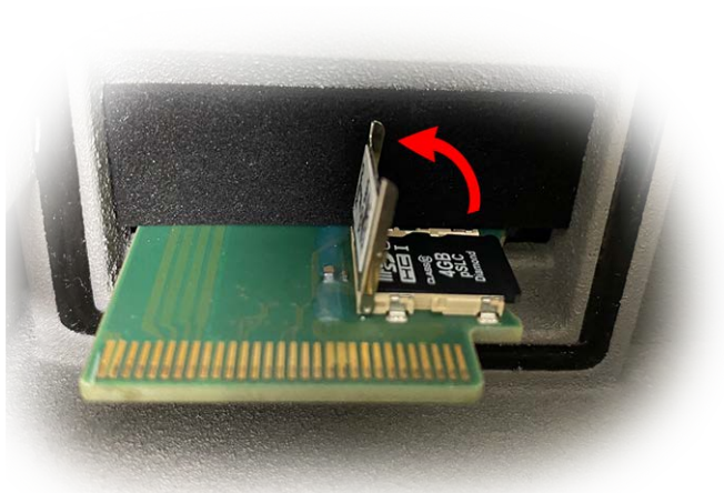
Abb. 96: Entriegeln des microSD-Kartenhalters
