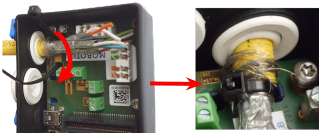
Abb. 58: Kabelbinder unter Netzwerkkabel eingeführt
