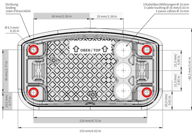
Abb. 31: Montageplatte mit Bohrungen zur Positionierung der Befestigungsschrauben
