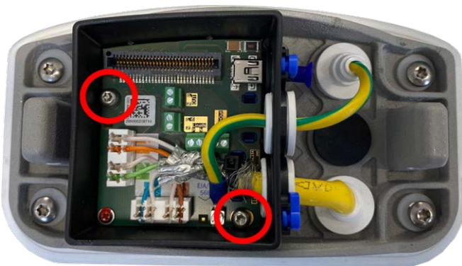
Abb. 64: Connector Box LSA (Draufsicht) mit zwei Schrauben (rot hervorgehoben) an Montageplatte montieren
