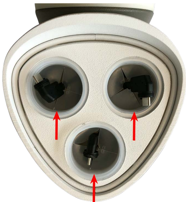
Abb. 8: Transportstopfen entfernen
