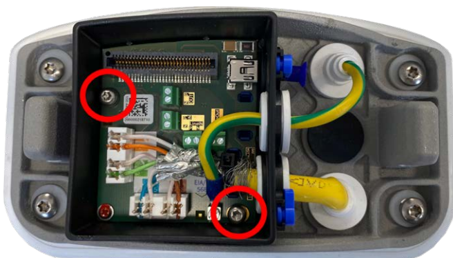
Fig. 64: Monte el Connector Box LSA (imagen superior) con los dos tornillos (resaltados en rojo) en la placa de montaje
