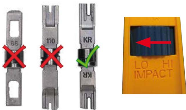
Fig. 59: Herramienta LSA+/Krone ajustada a un impacto BAJO
