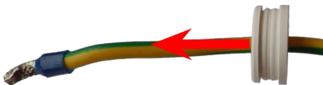
Fig. 61: Cable de tierra con tapón de caucho de un solo cable C.4
