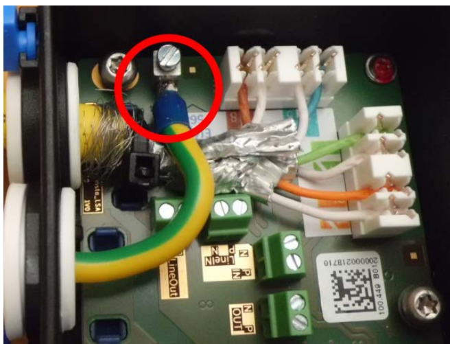
Fig. 63: Cable de tierra conectado al borne
