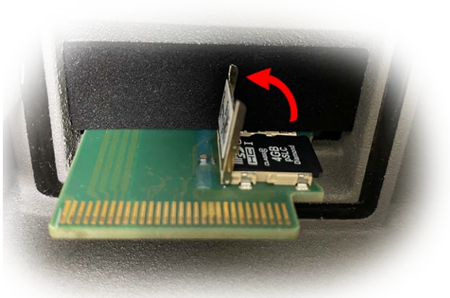
Fig. 96: Desbloquee el soporte de la tarjeta microSD
