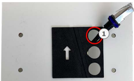
Fig. 44: Preparación de Connector Box RJ45
