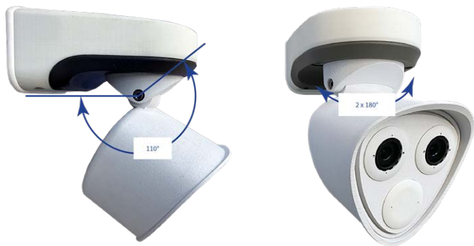
Fig. 30: Capacidad de inclinación cuando se monta en la pared
