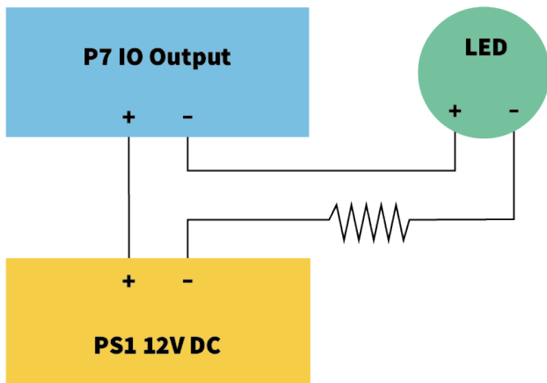
Fig. 68: Ejemplo: encendido de un LED
