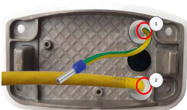
Fig. 36: Placa de montaje con cable de tierra y cable de red
