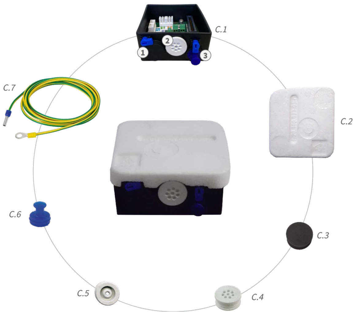
Fig. 3: Alcance de la entrega MOBOTIX M73 Connector Box LSA
