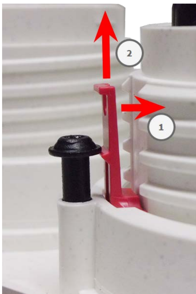
Fig. 20: Extracción de un clip de seguridad
