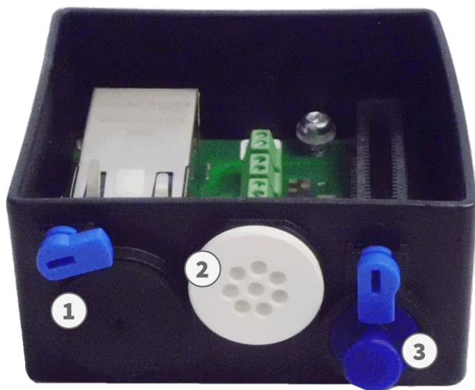
Fig. 65: Connector Box RJ45 con tapón de caucho negro C.3 ①, tapón de caucho de un solo cable C.4 ②, tapón para USB ③ y dos cierres azules
