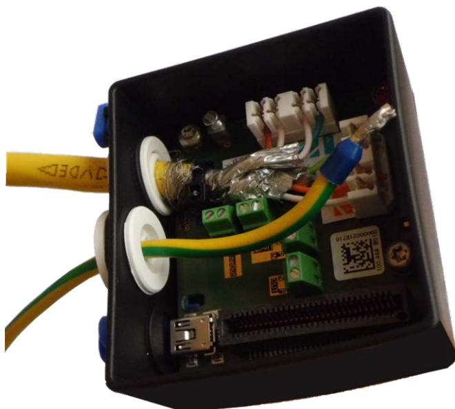
Fig. 62: El cable de tierra está introducido y tapón, correctamente colocado
