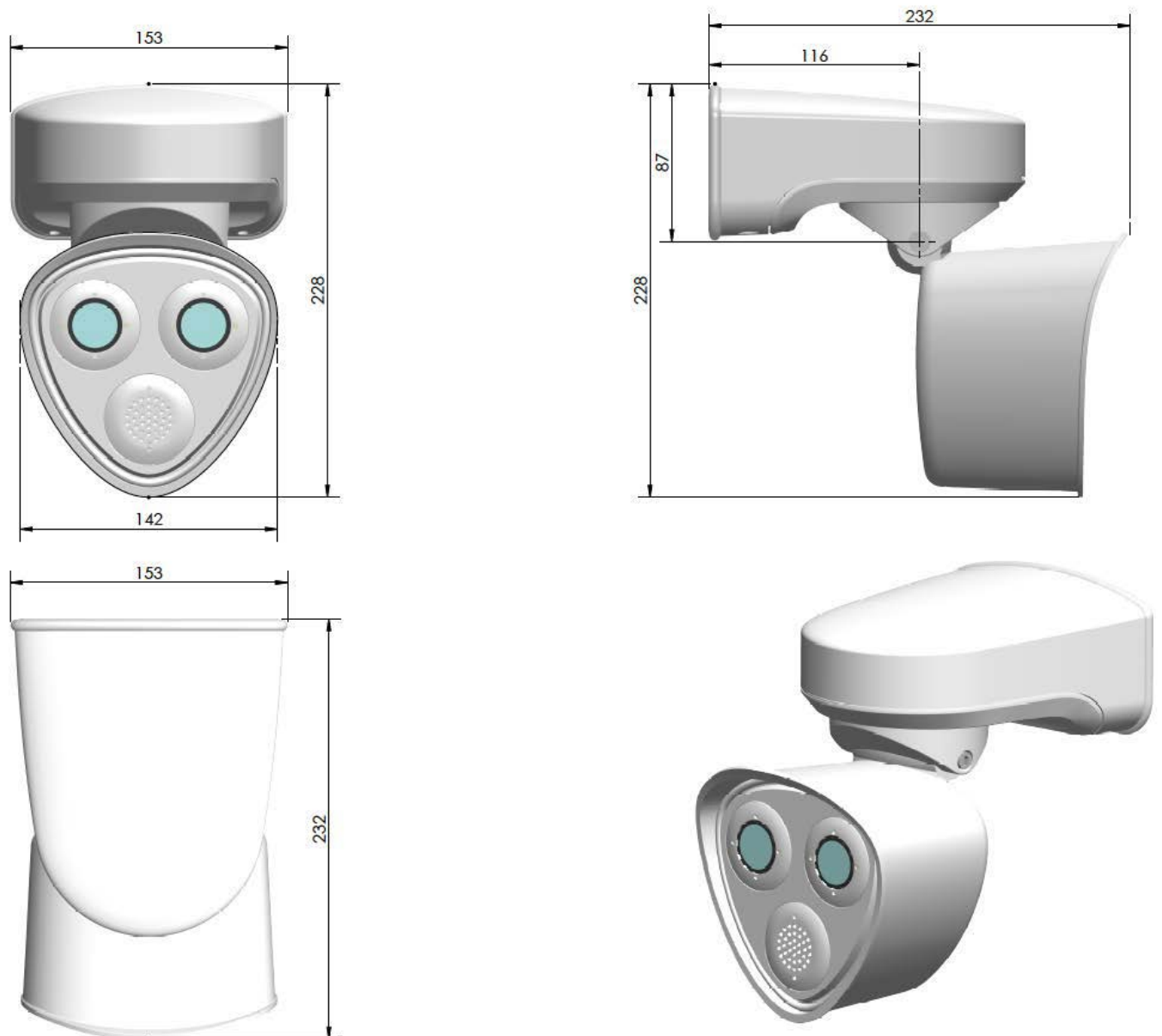
Fig. 5: MOBOTIX M73: Todas las medidas en mm
