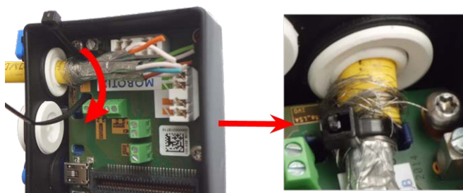
Fig. 58: Brida introducida debajo del cable de red
