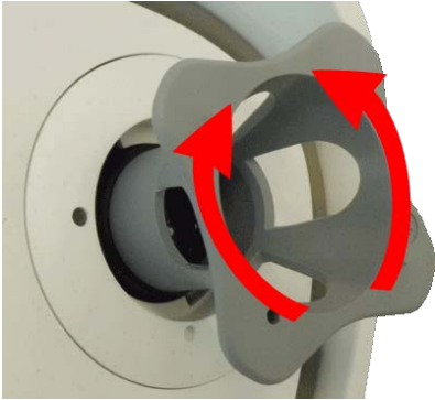
Fig. 85: Ajuste el enfoque del objetivo
