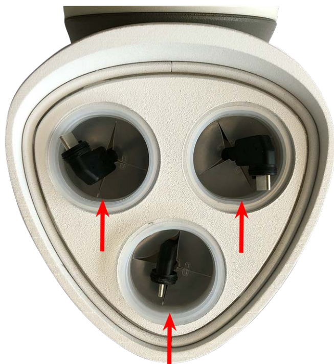
Fig. 8: Retire los tapones de transporte
