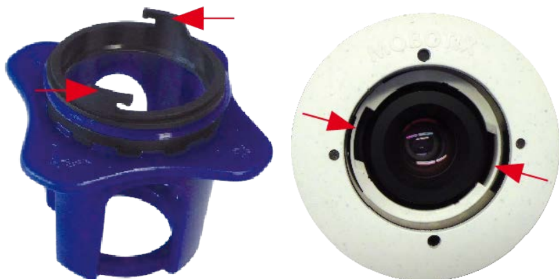
Fig. 87: Inserte el cristal de protección del objetivo con la llave de objetivo
