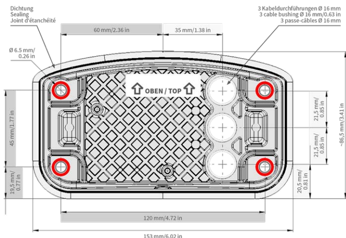
Fig. 31: Placa de montaje con agujeros para colocar los tornillos de fijación
