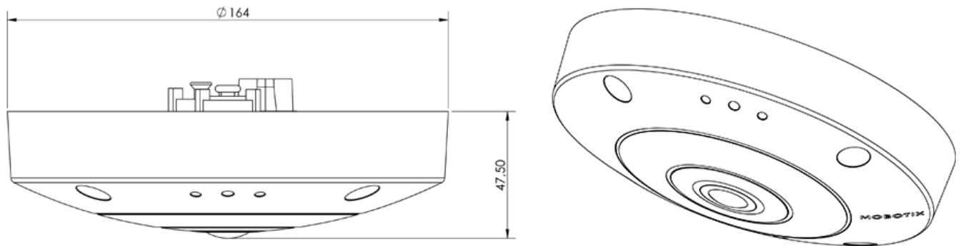
Abb. 5: MOBOTIX Q71: Alle Maßangaben in mm
