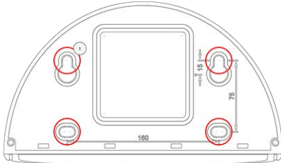
Abb. 8: Wall Mount mit Bohrungen zur Positionierung der Befestigungsschrauben
