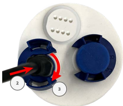
Abb. 16: Drücken Sie den Stecker fest ein, bis der blaue Dichtring einrastet.
