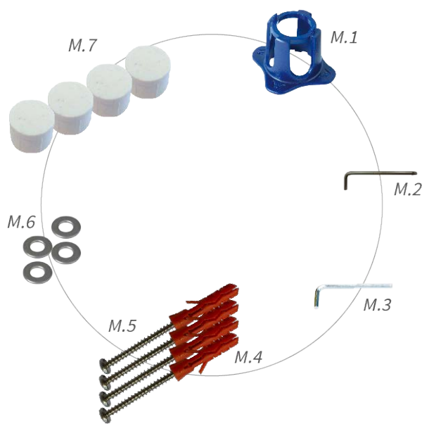
Fig. 2: Alcance de la entrega de los materiales de montaje MOBOTIX c71
