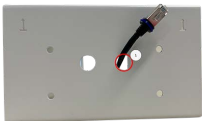
Fig. 12: Preparación del cableado de red
