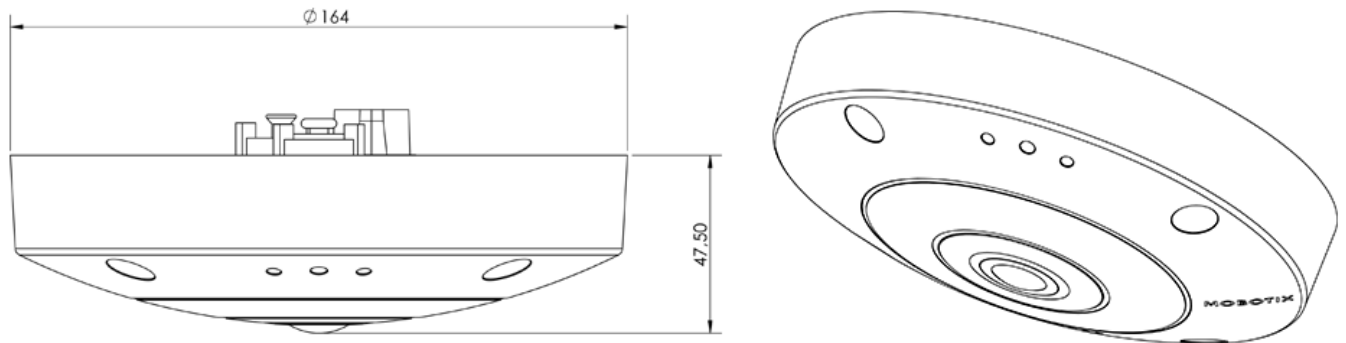
Fig. 5: MOBOTIX c71: Todas las medidas en mm
