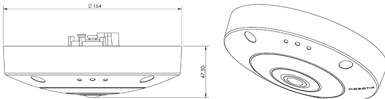
Fig. 5: MOBOTIX c71 : toutes les mesures sont en mm
