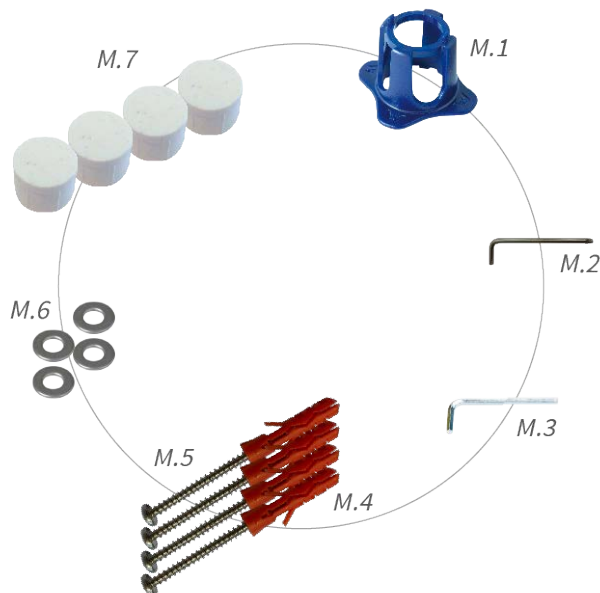
Fig. 2: Contenu de la livraison : accessoires de montage de MOBOTIX c71
