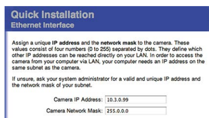
Fig. 21: Paramètres réseau dans l'interface Web de la caméra
