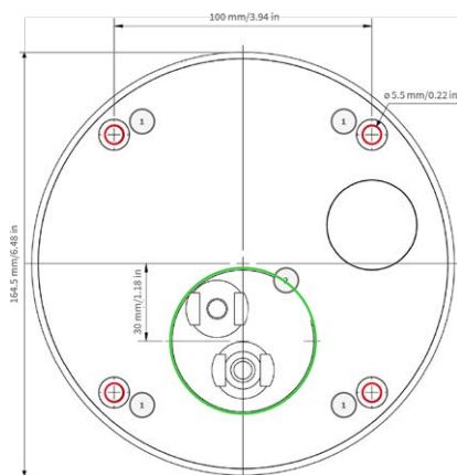
Fig. 7: Gabarit de perçage avec trous pour le positionnement des vis de fixation (cercles rouges) et pour la prise murale encastée (cercle vert)
