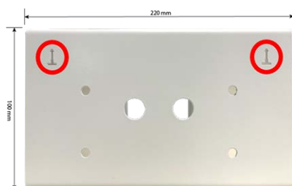
Fig. 10: Dimensions MOBOTIX p71 ECO Thermal Corner/Pole Mount – vue avant
