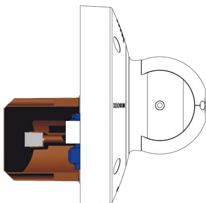
Fig. 6: Vue latérale de la MOBOTIX p71 ECO Thermal sur prise murale encastrée
