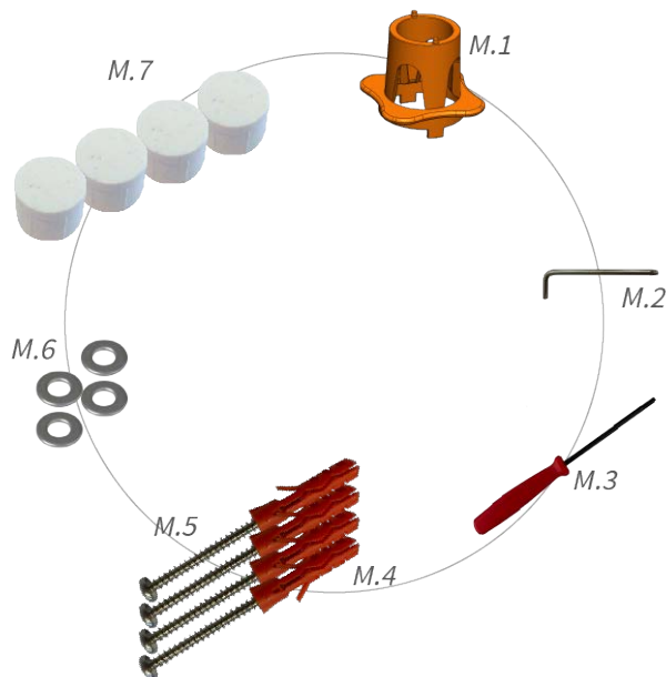
Fig. 2: Contenu de la livraison : accessoires de montage de MOBOTIX p71 ECO Thermal
