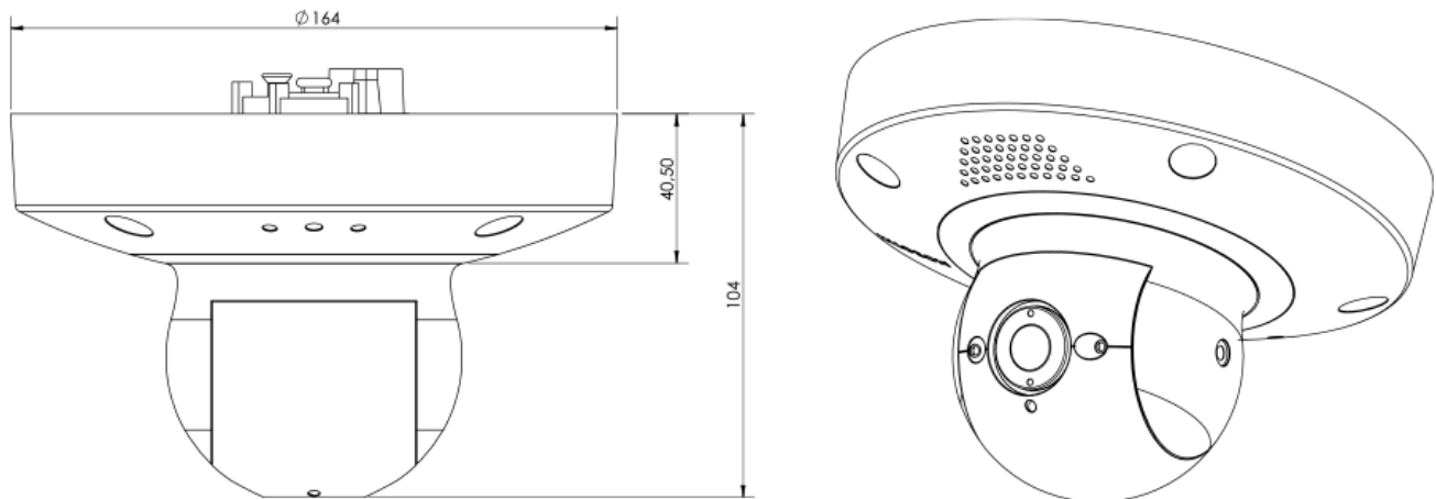
Abb. 5: MOBOTIX p71: Alle Maßangaben in mm
