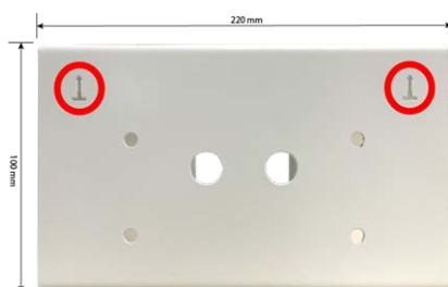
Abb. 10: Abmessungen MOBOTIX p71 Corner/Pole Mount – Vorderansicht
