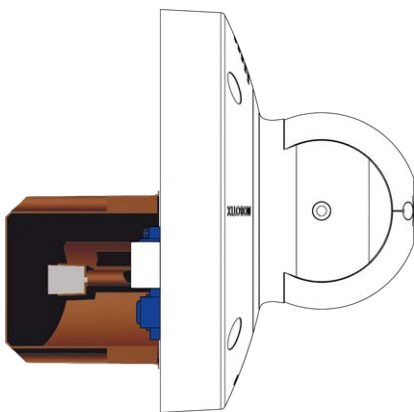
Abb. 6: Seitenansicht der MOBOTIX p71 über Unterputzsteckdose
