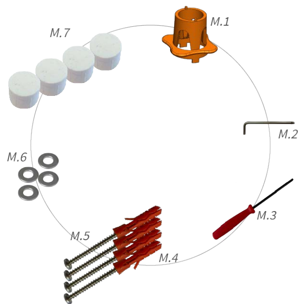
Abb. 2: Lieferumfang MOBOTIX p71 Montagezubehör
