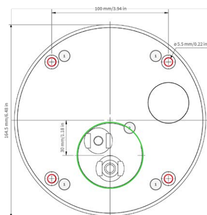
Fig. 7: Dima di foratura con fori per il posizionamento delle viti di fissaggio (cerchi rossi) e per la presa a muro a incasso (cerchio verde)
