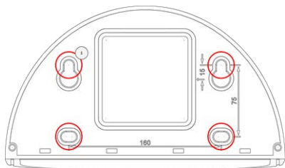
Fig. 8: Wall Mount con fori per il posizionamento delle viti di fissaggio
