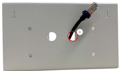
Fig. 15: Preparare il cablaggio di rete
