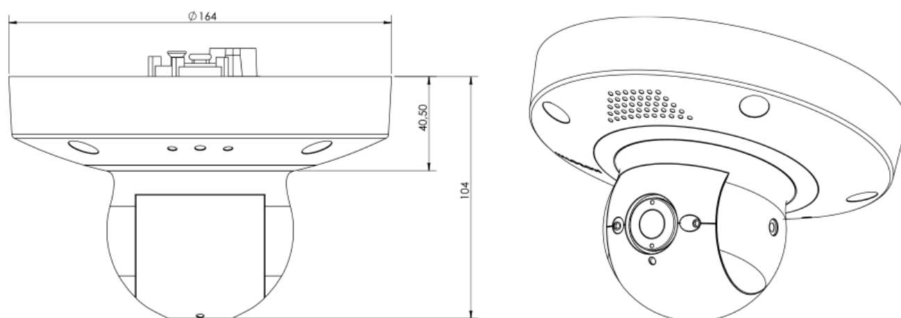
Fig. 5: MOBOTIX p71: Tutte le misurazioni in mm
