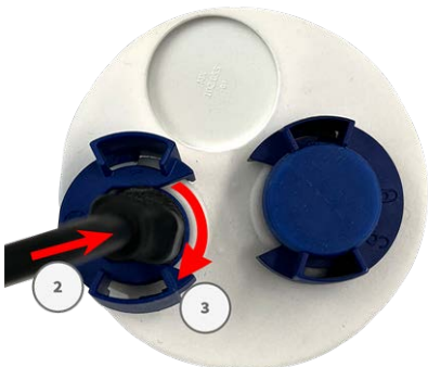
Fig. 16: Premere con decisione il tappo fino a quando l'anello di tenuta blu non scatta in posizione
