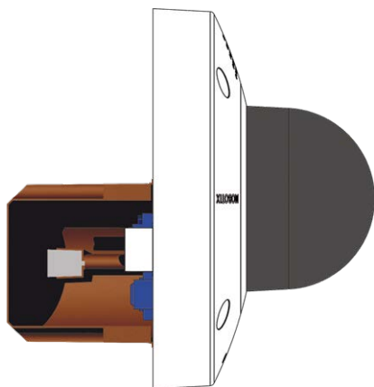
Fig. 6: Vue latérale de la MOBOTIX v71 sur prise murale encastrée
