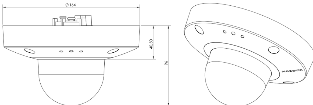
Fig. 5: MOBOTIX v71 : toutes les mesures sont en mm
