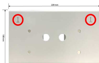
Fig. 10: Dimensions MOBOTIX v71 Corner/Pole Mount – vue avant
