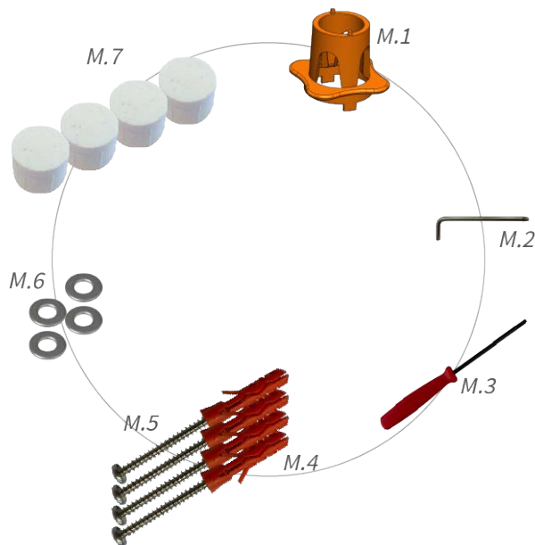
Fig. 2: Contenuto della confezione MOBOTIX v71 Materiali di montaggio
