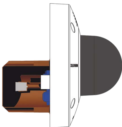
Fig. 6: Vista laterale di MOBOTIX v71 con presa a muro a incasso
