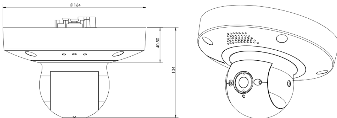
Fig. 1: MOBOTIX p71 ECO Thermal: Tutte le misurazioni in mm
