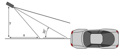
Fig. 11: Alineación horizontal de la cámara
