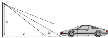
Fig. 10: Orientación vertical de la cámara
