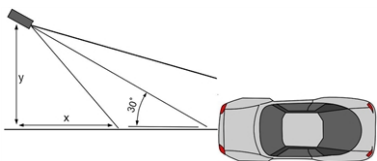
Fig. 11: Alineación horizontal de la cámara
