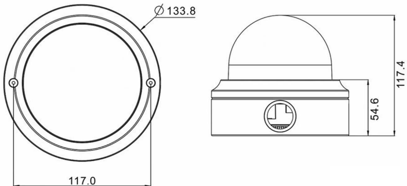
Abb. 1: 2MP Vandal Fixed Dome Analytics Camera: Alle Maßangaben in mm
