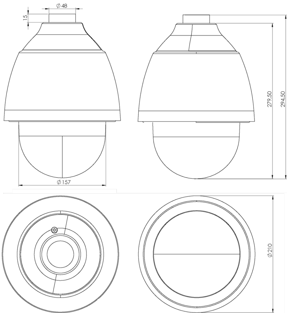
Fig. 1: 2MP Low-Light Video Analytics Speed Dome: Tutte le misure sono espresse in mm
